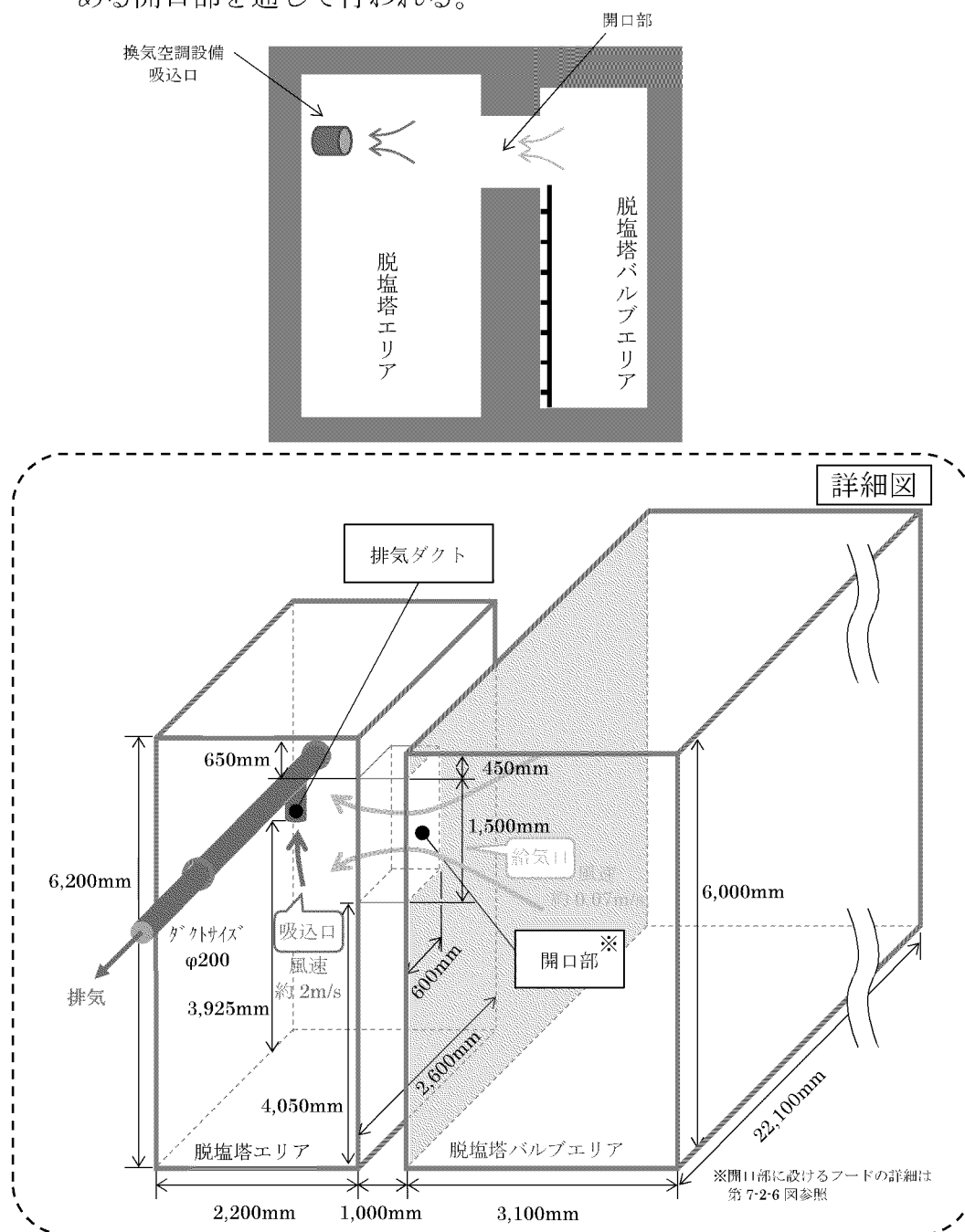
第 7-2-5 図 脱塩塔エリアの詳細図 (例：A 使用済燃料ピット脱塩塔エリア)
