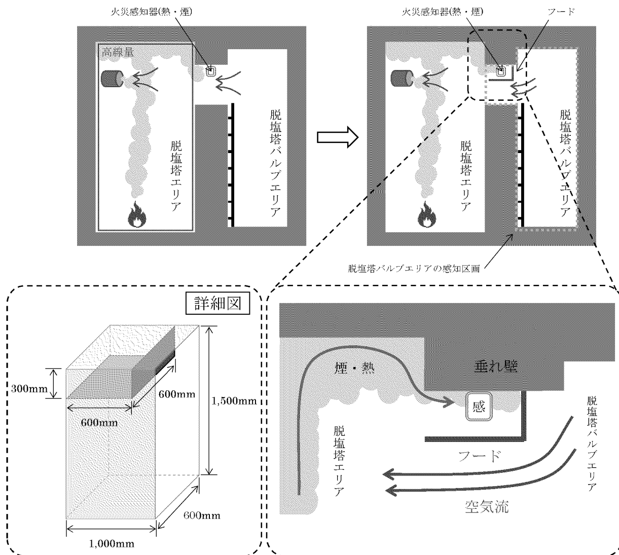
第 7-2-6 図 脱塩塔エリア開口部におけるフードを用いた火災感知器の設置概要
