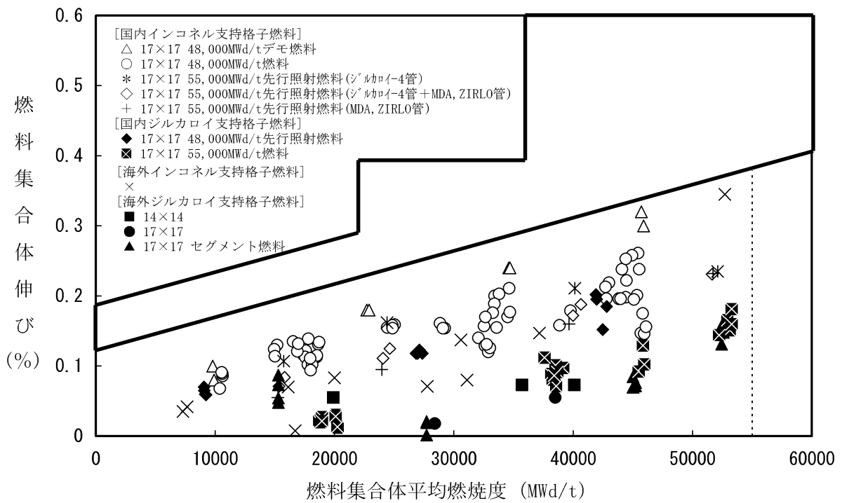
図 3-14 燃料集合体伸び (5) ~ (10)
