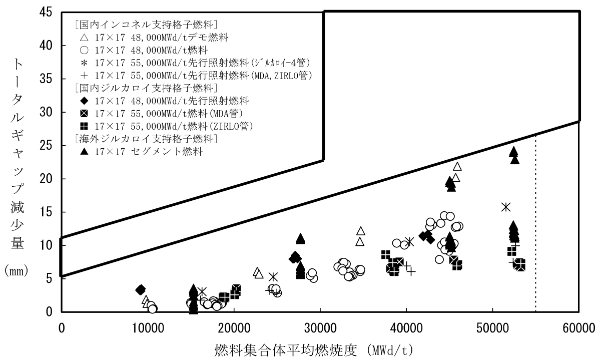
図 3-15 トータルギャップ減少量 (5)、(6)
