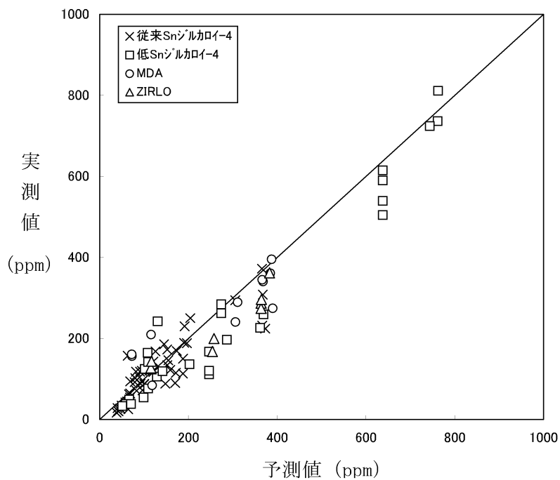
図 3-17 被覆管水素吸収量の実測値と予測値の比較 (12)
