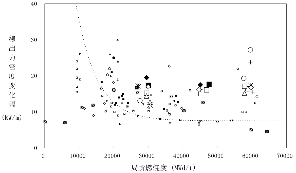
図 3-18 (2) 被覆管の出力ランプ試験結果 (6)、(13)～(15) (線出力密度変化幅が最大の場合の出力変化)
