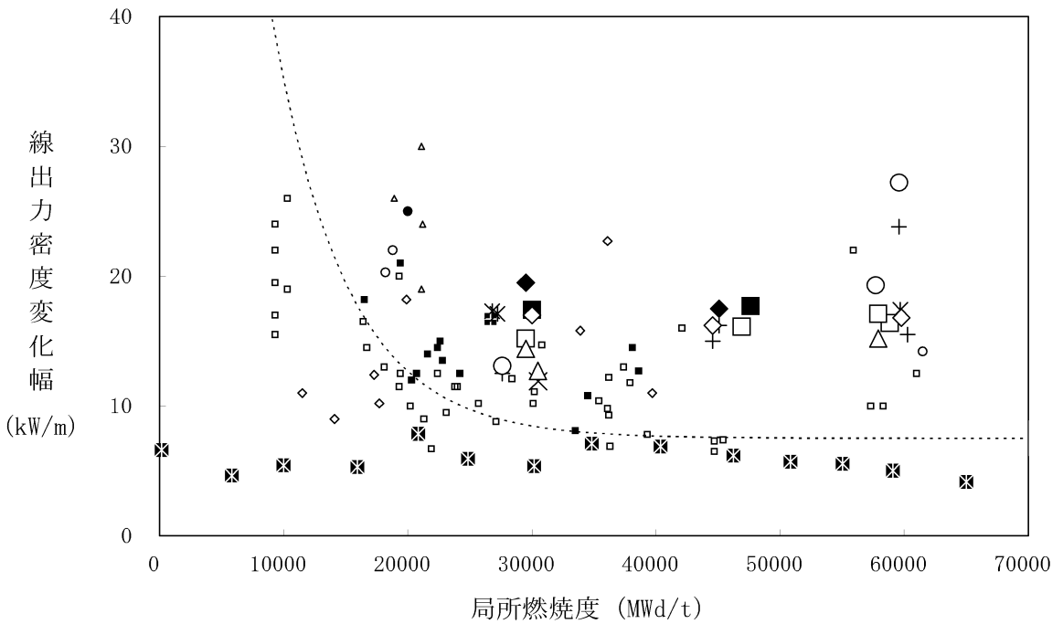
図 3-18 (1) 被覆管の出力ランプ試験結果 (6)、(13)～(15) (最大線出力密度が最大の場合の出力変化)
