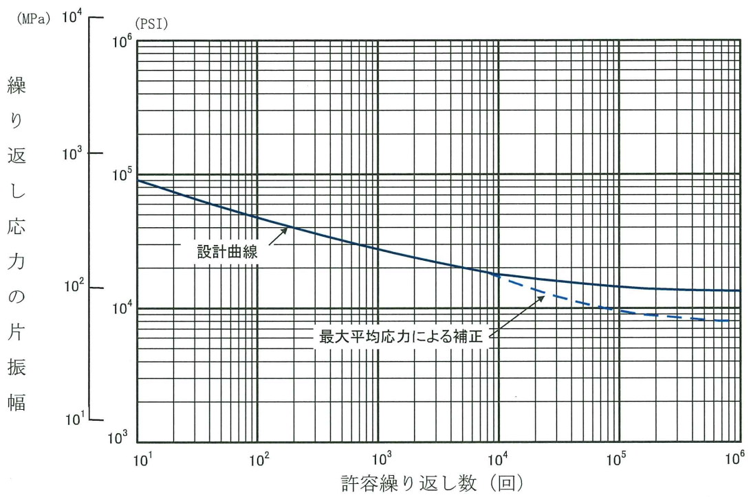
図 3-7 ジルカロイ-4 の設計疲労曲線 (2)
