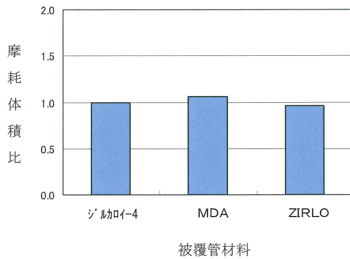
図 3-20 ジルカロイ-4 支持格子との組合せにおける被覆管材料の摩耗体積比の比較
