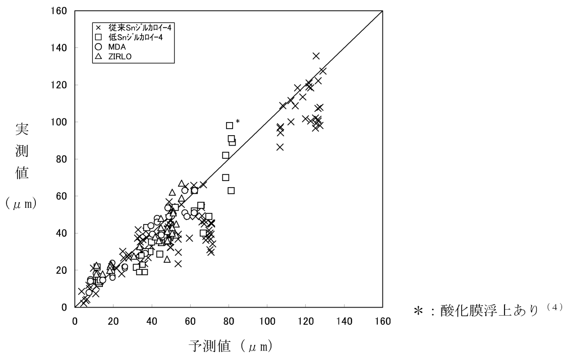
図 3-16 被覆管腐食量 (最大酸化膜厚) の実測値と予測値の比較 (11) 、 (12)
