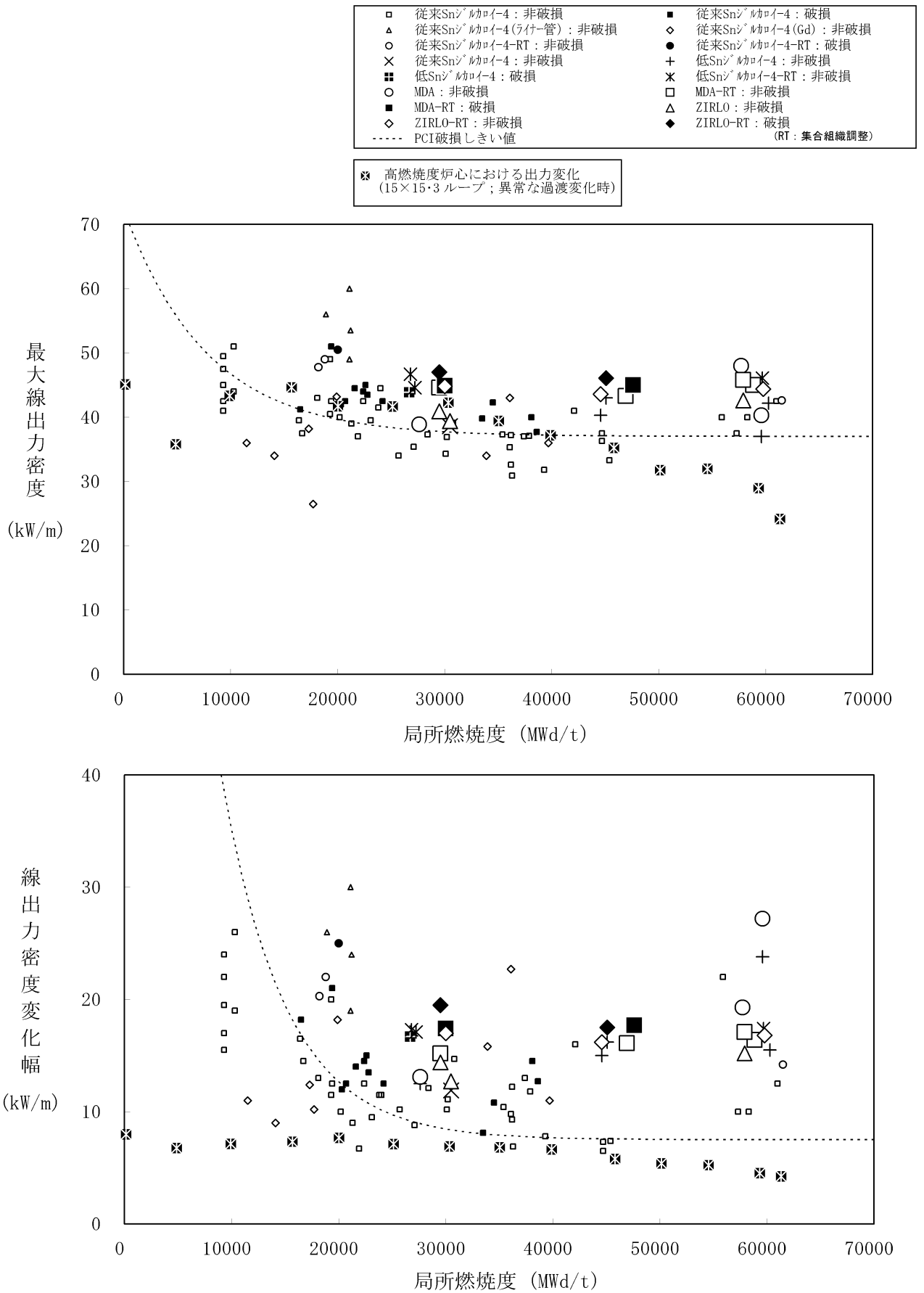
図 3-18 (1) 被覆管の出力ランプ試験結果 (7)~(10) (最大線出力密度が最大の場合の出力変化)
