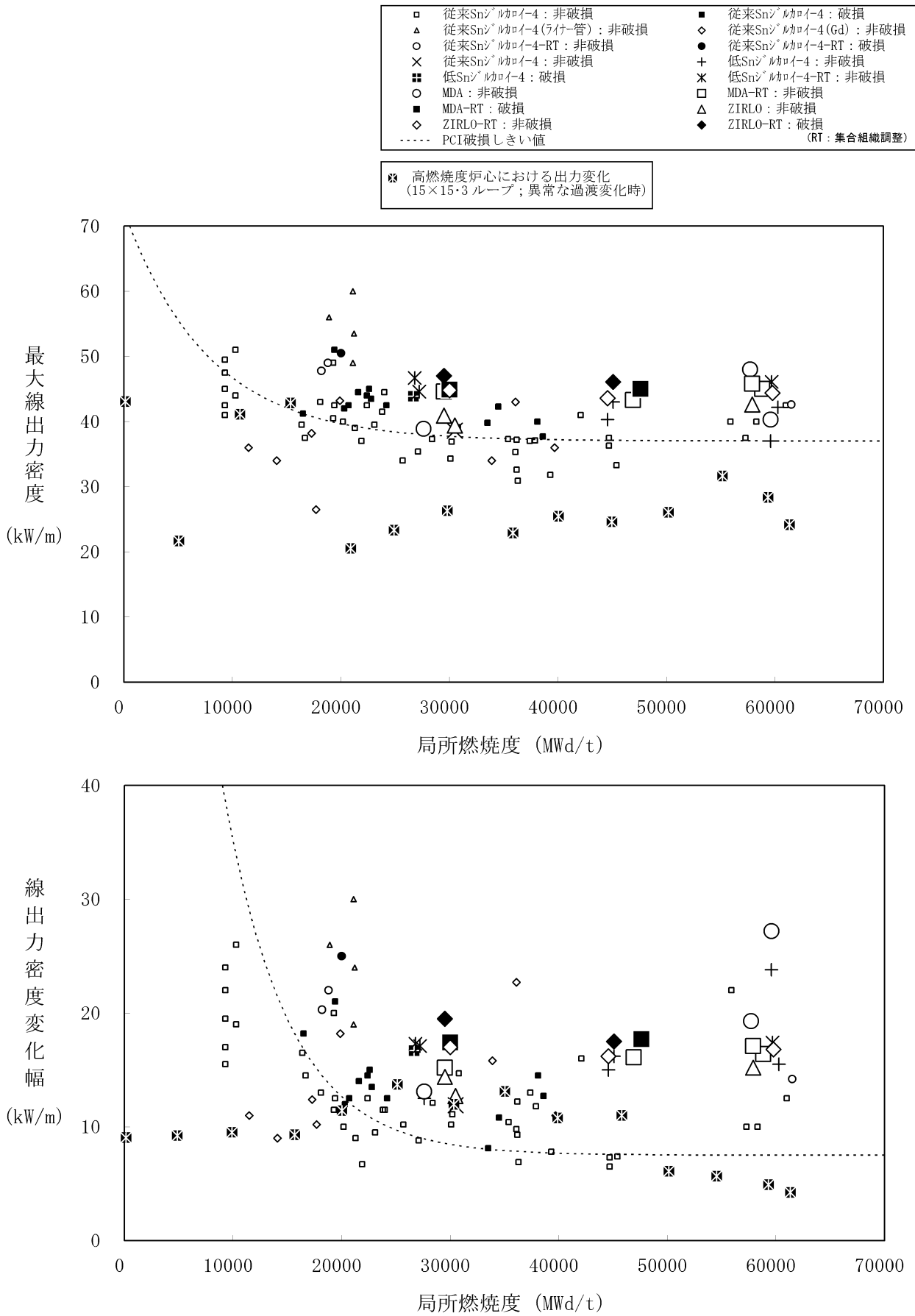
図 3-18 (2) 被覆管の出力ランプ試験結果 (7)~(10) (線出力密度変化幅が最大の場合の出力変化)
