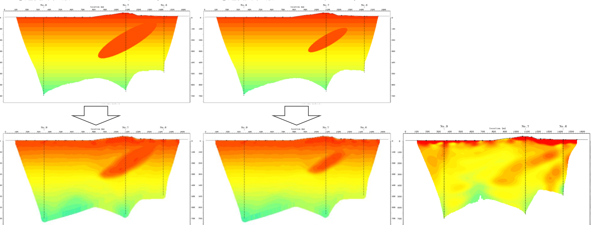
S波の初動解析結果（6-7-9測線）
