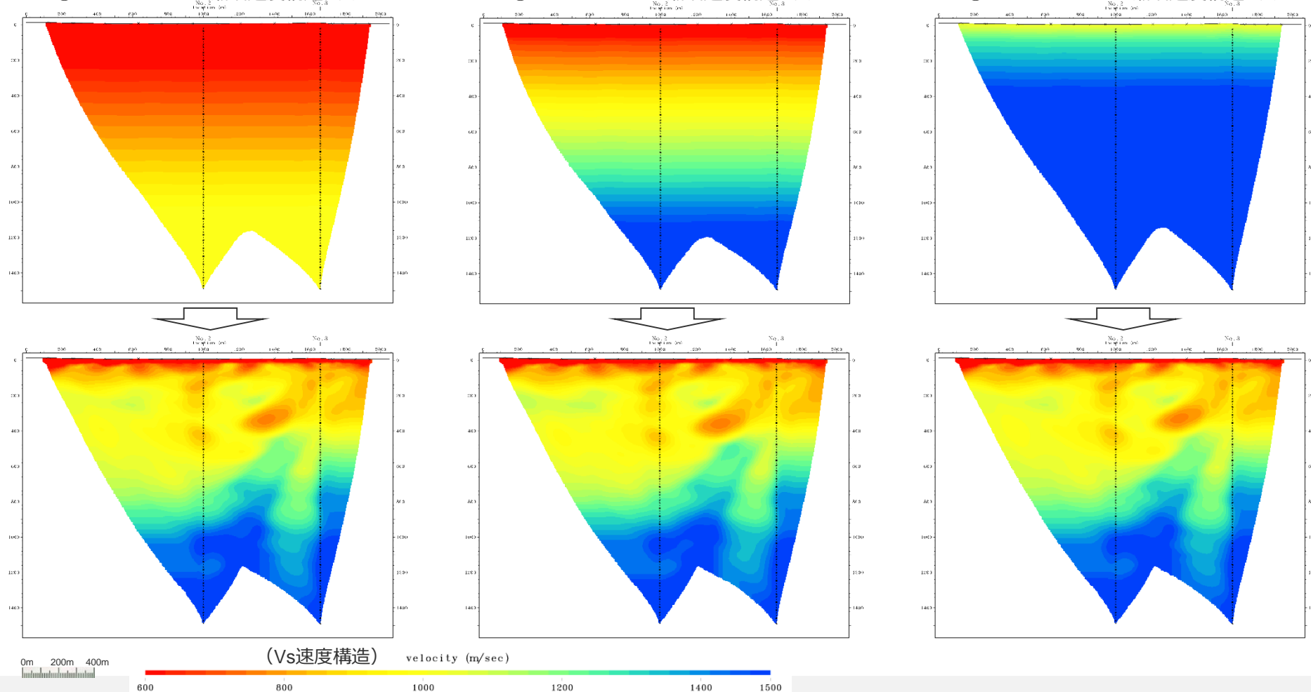
①400～1000m/sの漸増速度構造モデル
