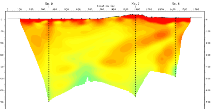
S波の初動解析結果（6-7-9測線）
