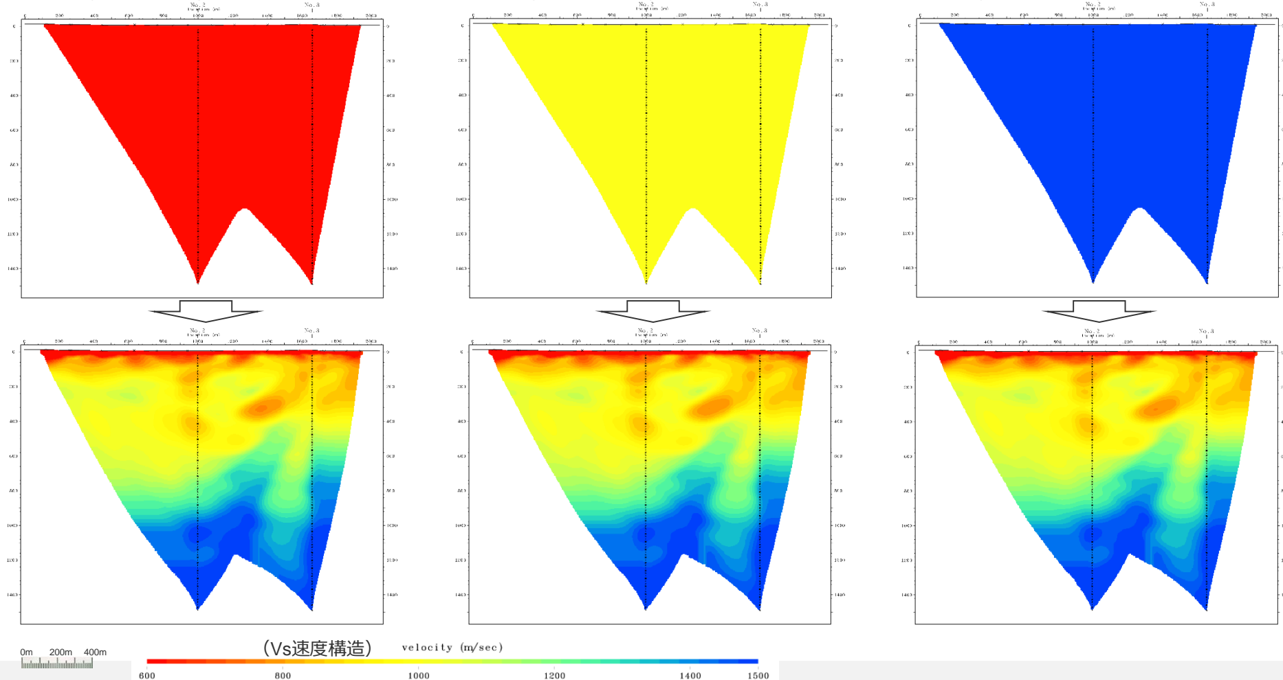
①500m/sの一様速度構造モデル
