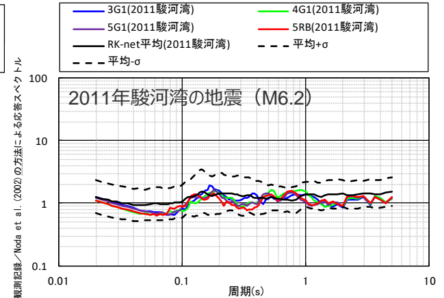
<地震観測記録とNoda et al.(2002)の方法による応答スペクトルの比 (水平平均) >
