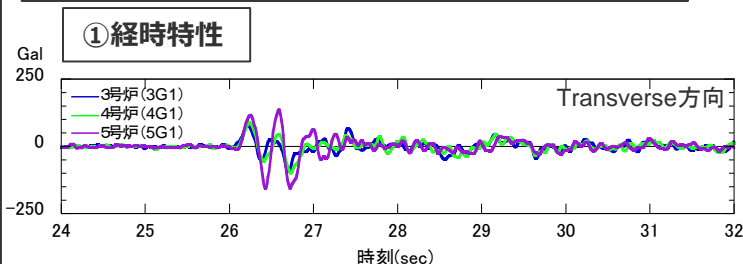
<2009年駿河湾の地震（本震）の加速度時刻歴波形>
