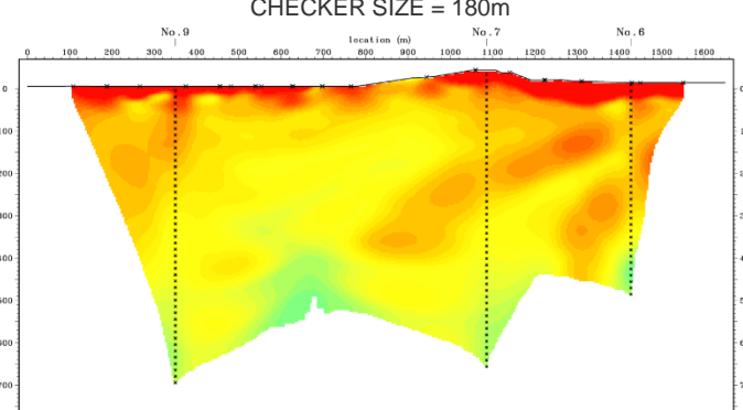
S波の初動解析結果（6-7-9測線）
