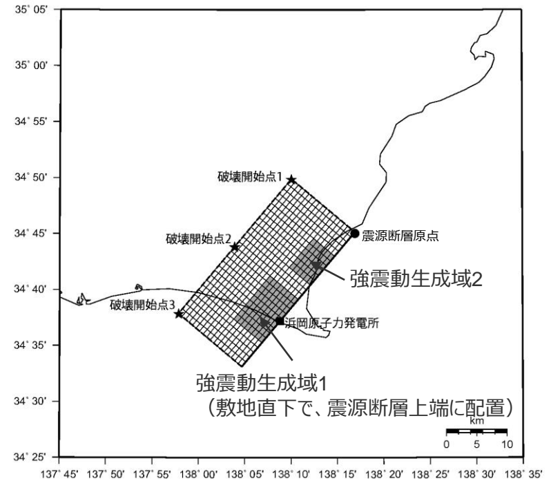
<基本震源モデル（地震動の顕著な増幅を考慮しない） （敷地下方の想定スラブ内地震）>
