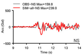
電中研御前崎 (CRIEPI-OMZ)
