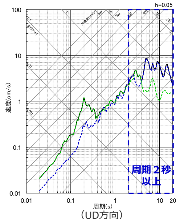
— 全体波形 — 40～90秒波形 — 0～40秒波形
