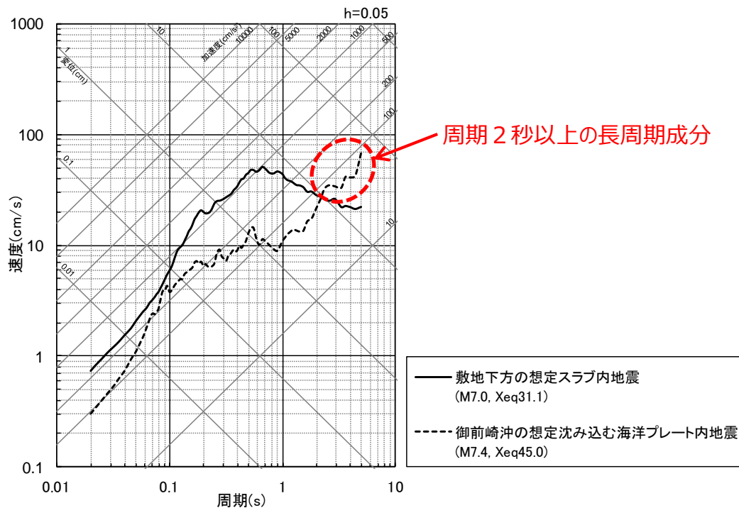
<Noda et al.(2002)の方法による地震動評価結果の比較>
