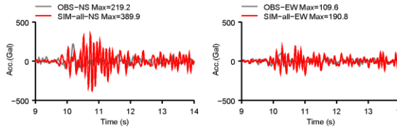
K-NET土肥 (SZO006)
