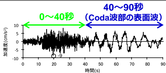
— 全体波形 — 40～90秒波形 — 0～40秒波形
