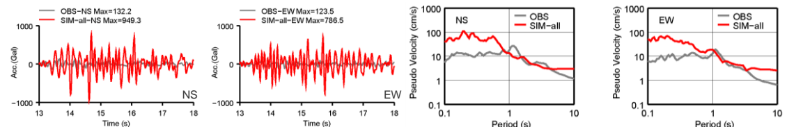
K-NET沼津 (SZO008)
