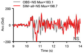
地震研御前崎 (ERI-OMZ)
