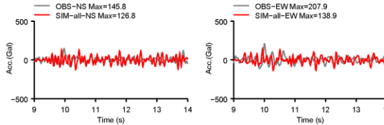
K-NET西伊豆 (SZO027)
