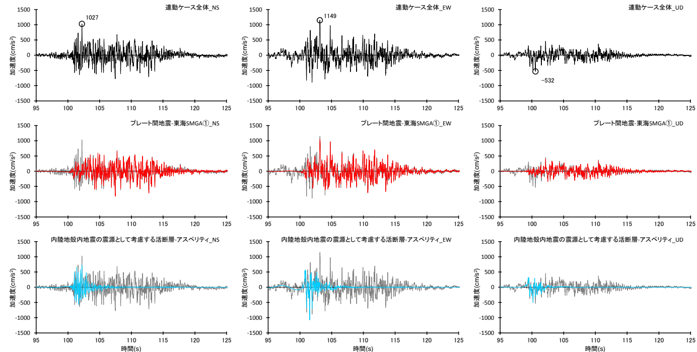
<連動ケース全体、プレート間地震の東海SMGA①、内陸地殻内地震の震源として考慮する活断層のアスペリティの加速度時刻歴波形の比較>
