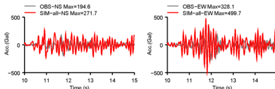
K-NET南伊豆 (SZO004)
