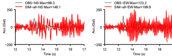
K-NET修善寺 (SZO007)
