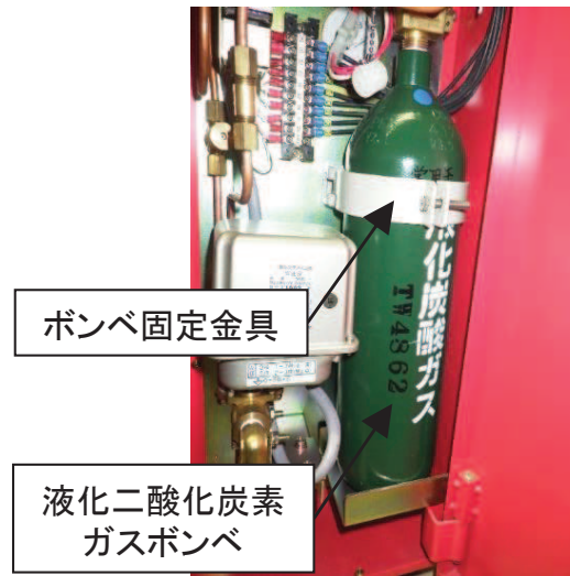
図17 発電所におけるボンベの設置状況
