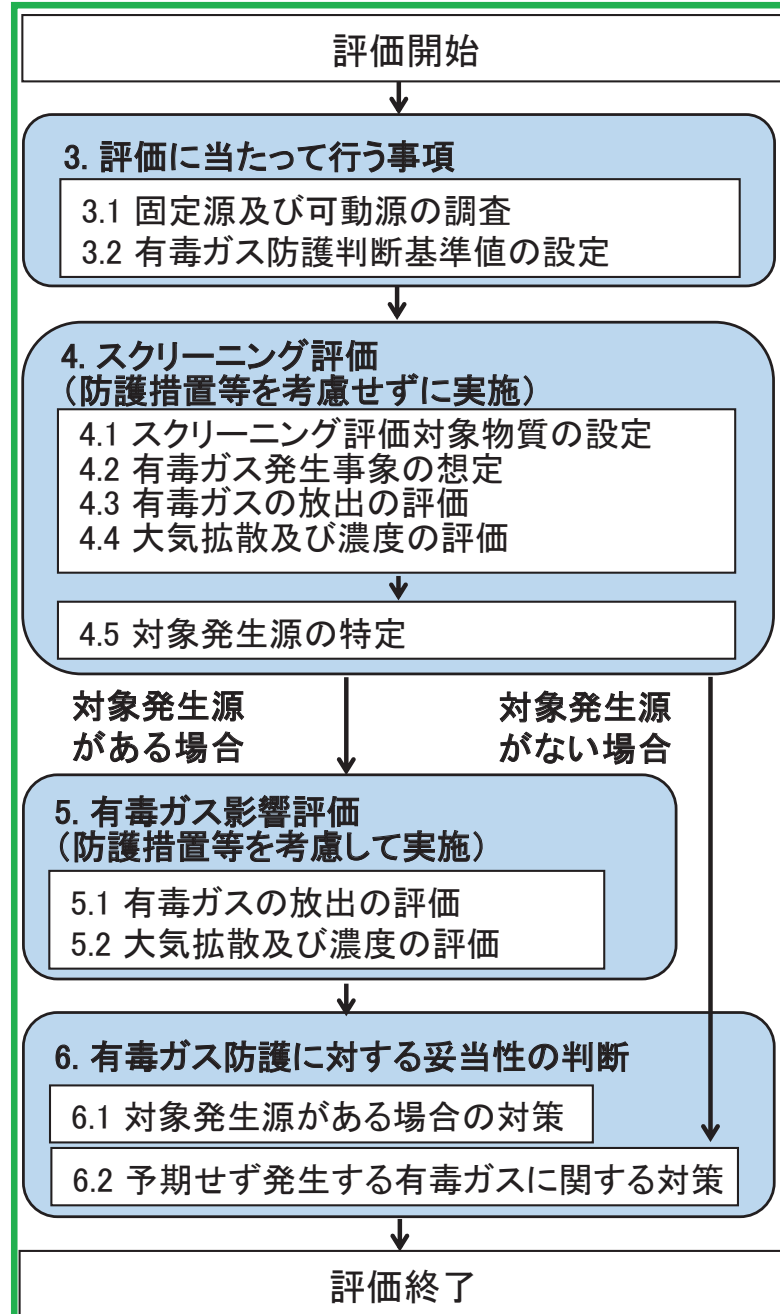
図1 有毒ガス防護に係る妥当性確認の流れ (ガイド2.のとおり)
