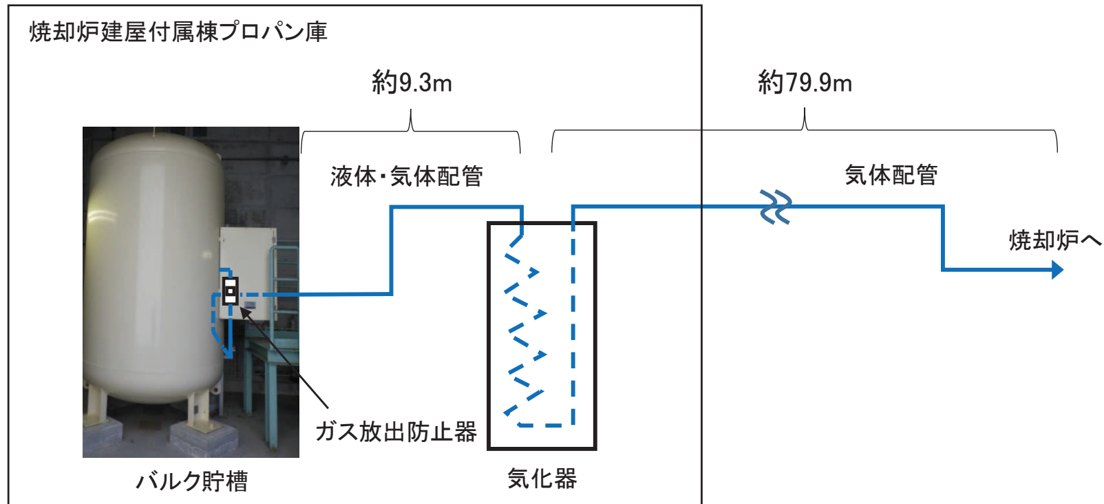
図18 廃棄物焼却設備のプロパンガス概略系統図
