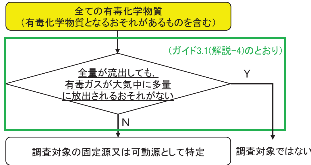
図4 調査対象の固定源又は可動源の特定フロー
