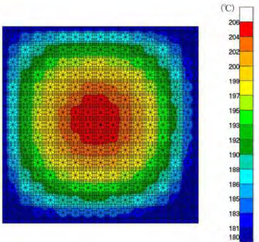
(15×15燃料収納時)
