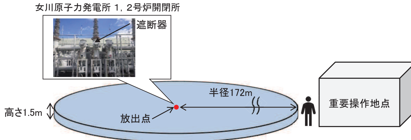
図24 六フッ化硫黄と評価地点の関係
