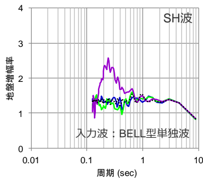
<地盤増幅率>
