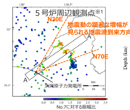
<各地震の振幅比 (No.7基準) の震央分布図>
