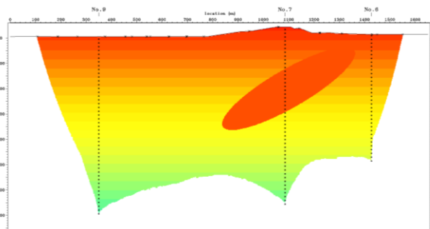
①速度異常域が600m×150m（700m/s）のモデル
