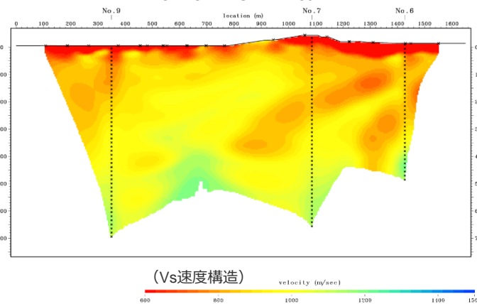
S波の初動解析結果（6-7-9測線）
