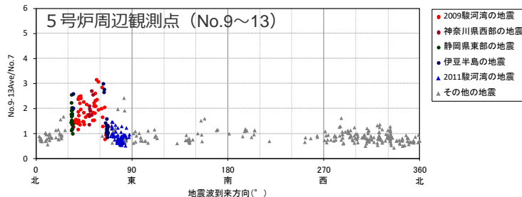
<地震波到来方向毎の振幅比（No.7基準）（水平平均）>
