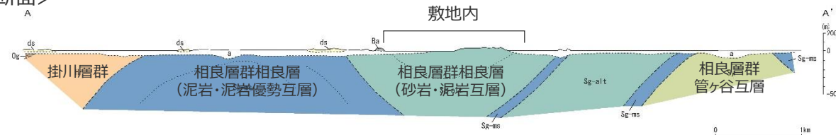
<反射断面 (Line3) >
