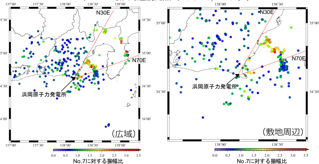
(5号炉周辺観測点 (No.9~13)) <各地震の振幅比 (No.7基準) の震央分布図>
