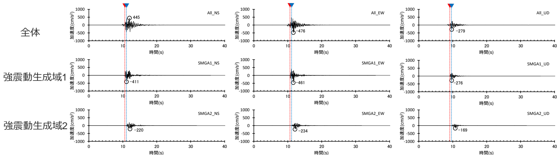
<ケーススタディモデル④の加速度時刻歴波形>
