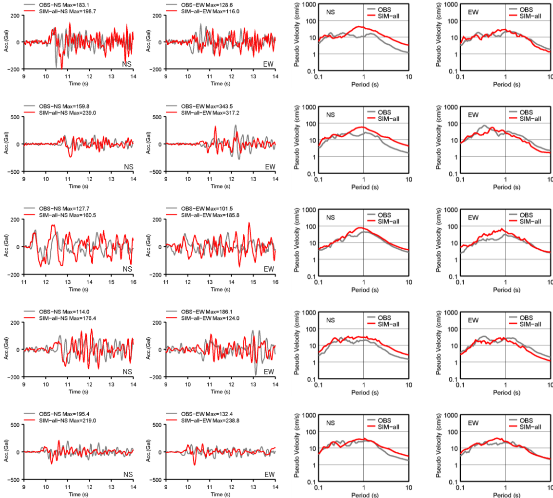
<経験的グリーン関数法によるシミュレーション結果と観測記録との比較（敷地周辺）> (左図：加速度時刻歴波形、右図：応答スペクトル)
