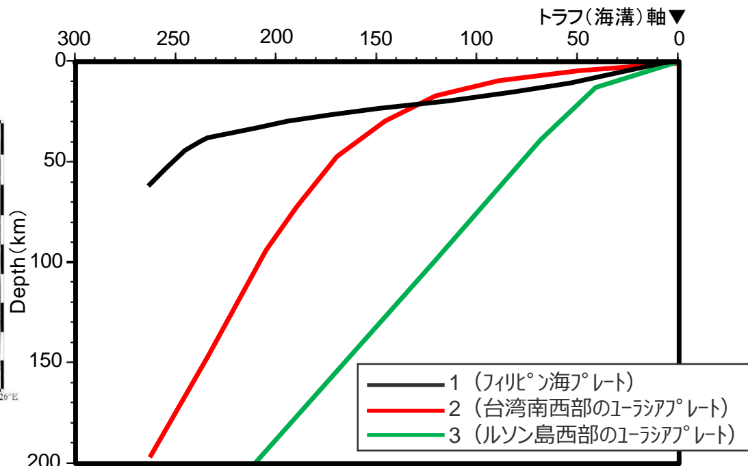
<海洋プレートの沈み込み断面図>
