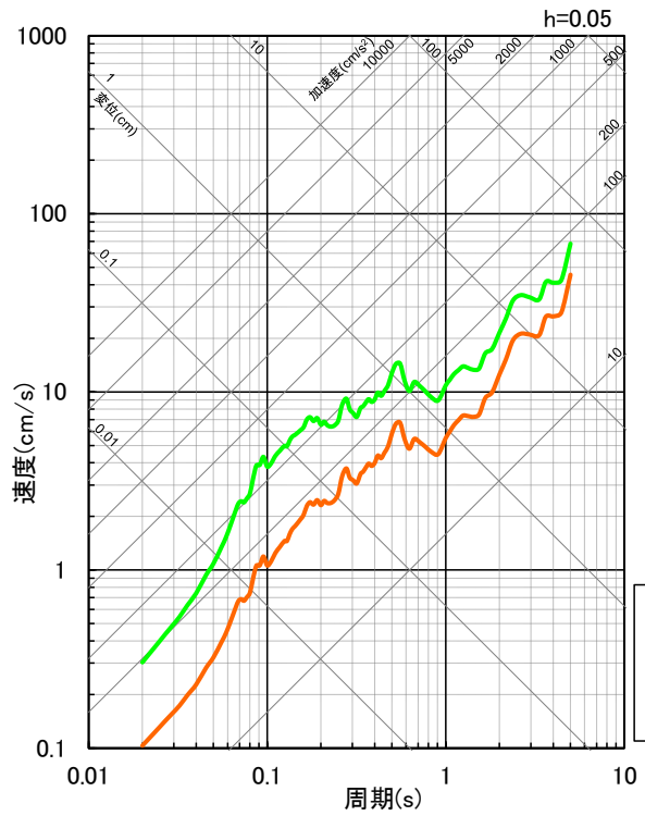
<Noda et al.(2002)の方法による地震動評価結果の比較>
