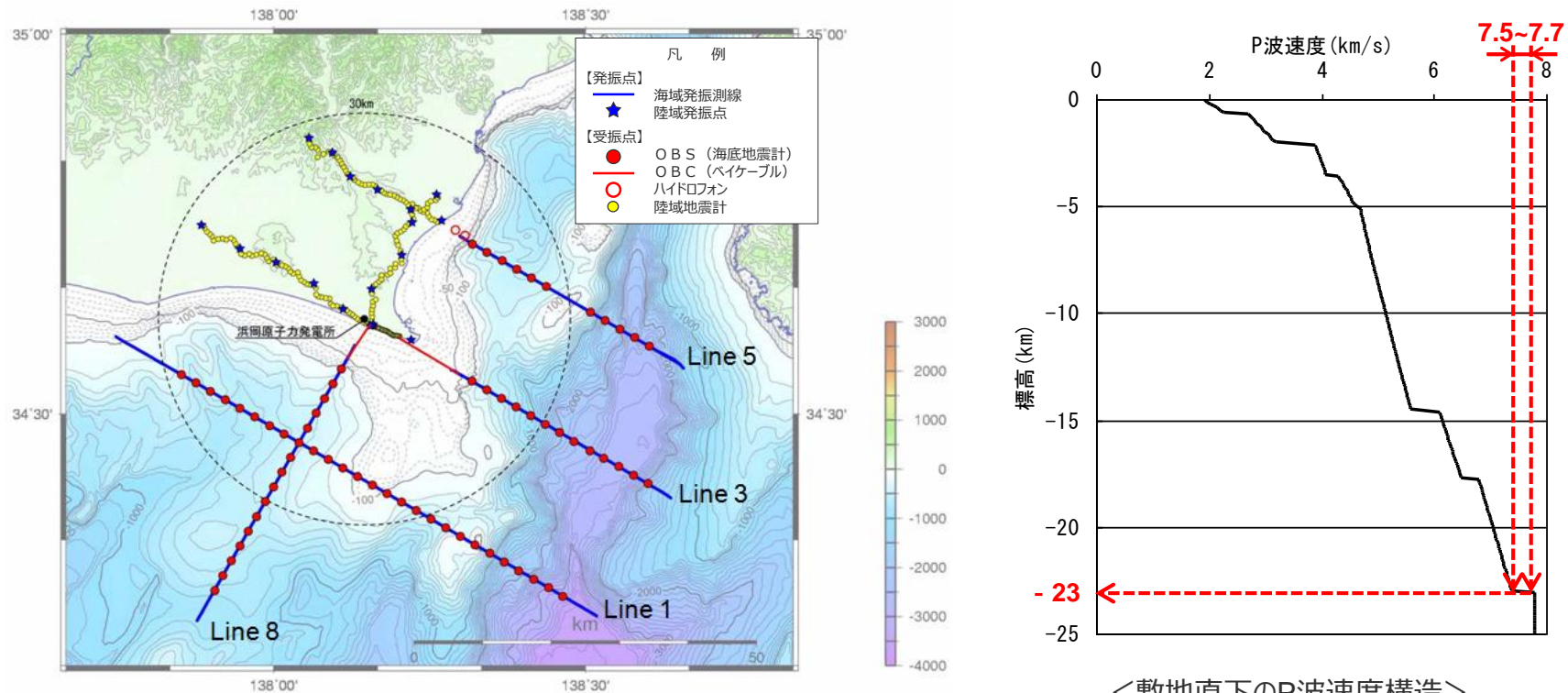
<屈折法地震探査（Line1, 3, 5, 8）の測線>
