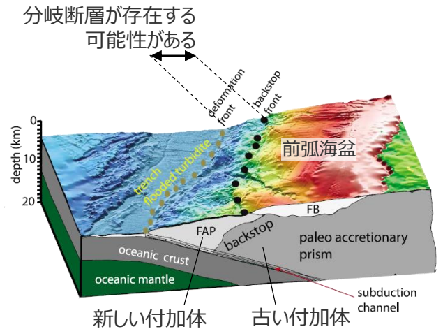
<チリの分岐断層の地形> (Contreras-Reyes et al.(2010)に図の説明 (前弧海盆、新しい付加体、古い付加体)、分岐断層が存在する可能性がある旨を加筆)
