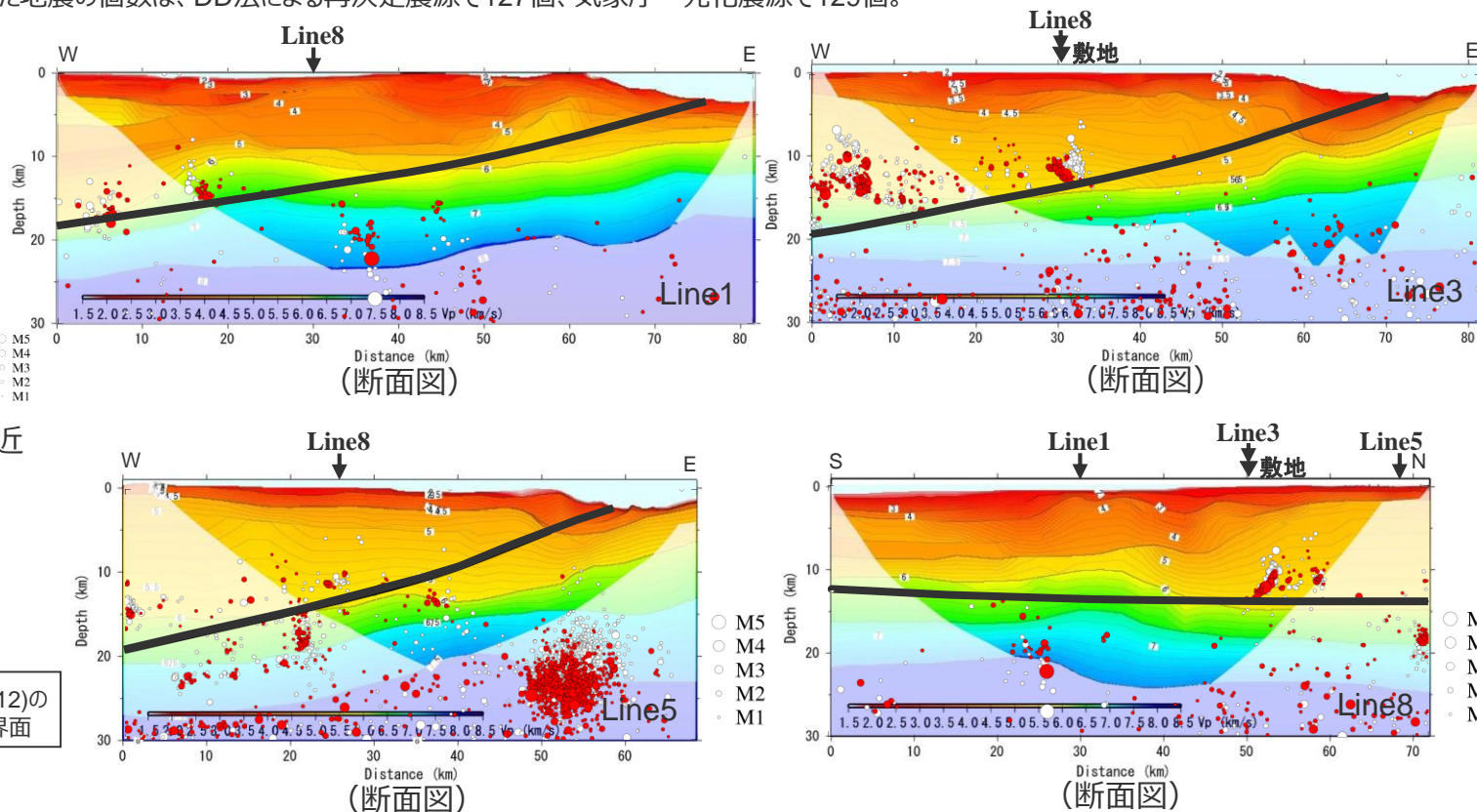
<屈折法地震探査によるP波速度構造 (Line1,3,5,8) と震源鉛直分布> (観測分析期間: 1997年10月~2015年12月)
