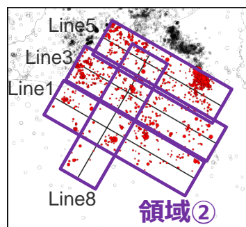
(屈折法地震探査の測線付近で発生した地震の震央分布)
