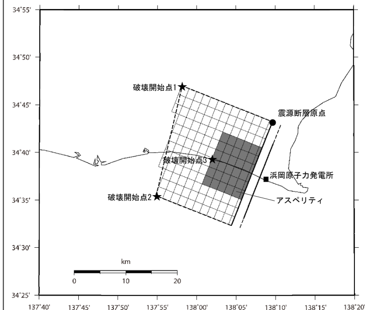
<基本震源モデル（地震動の顕著な増幅を考慮しない） （A-17断層による地震）※3>
