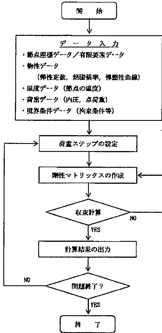
図 3.5-1 ABAQUS コードの解析フロー図
