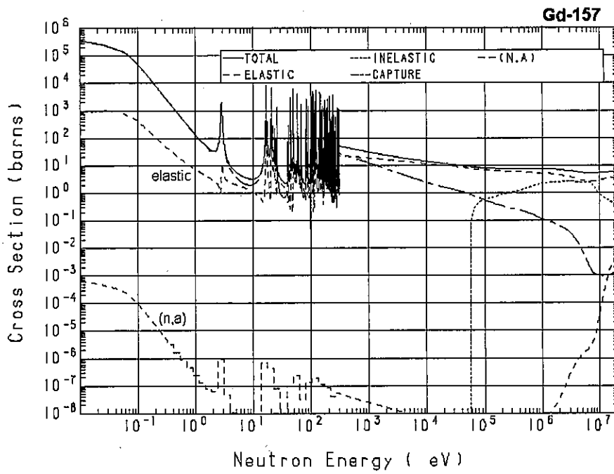
Gd-157 の反応断面積
