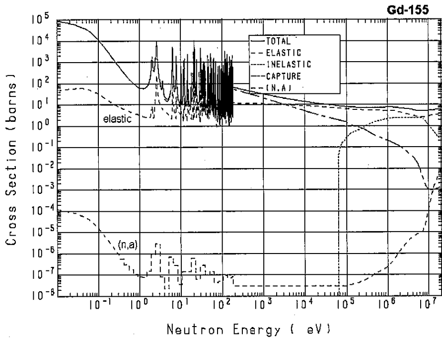
Gd-155 の反応断面積
