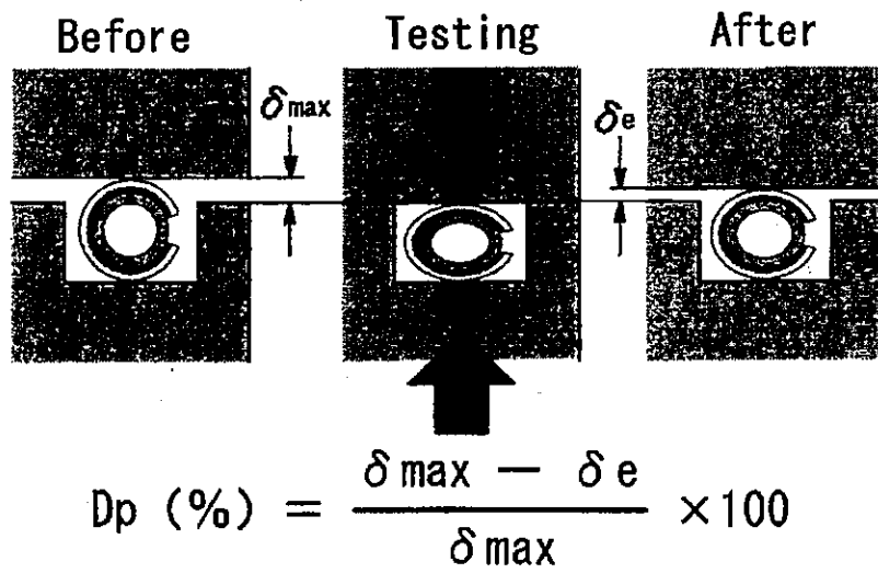
図 1-13 塑性変形率の定義 (17)
