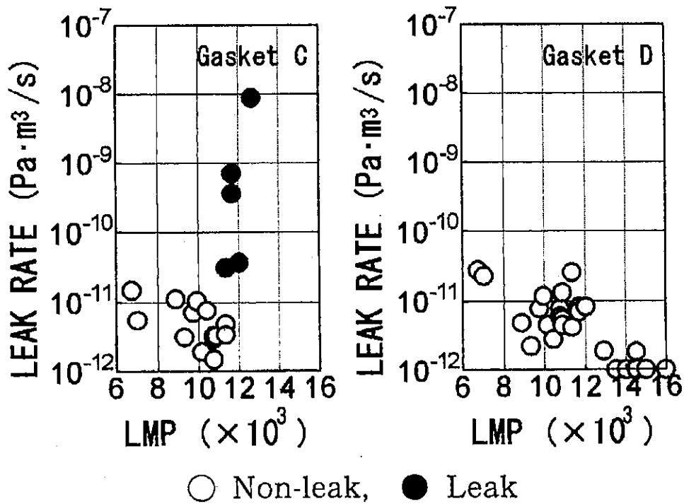
図 1-14 漏えい率と LMP の関係 (17)
