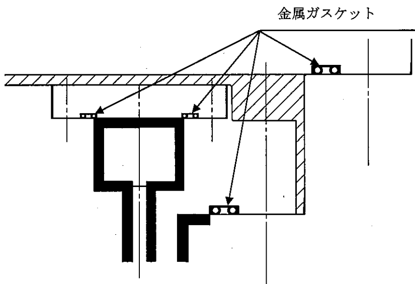
A部詳細
