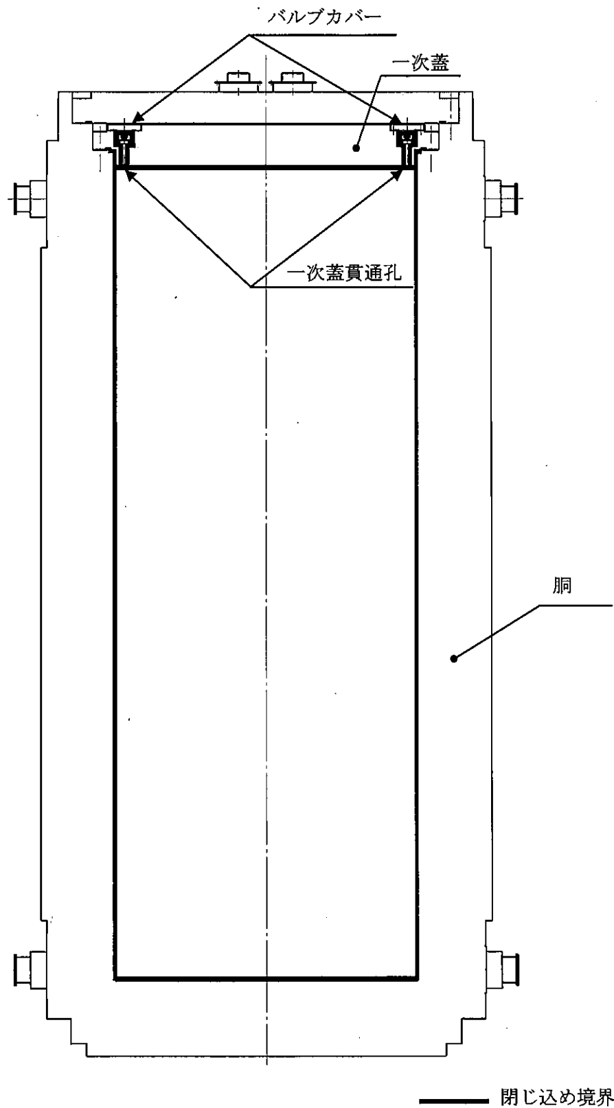
図 1-7 HDP-69BCH(B)型の閉じ込め構造
