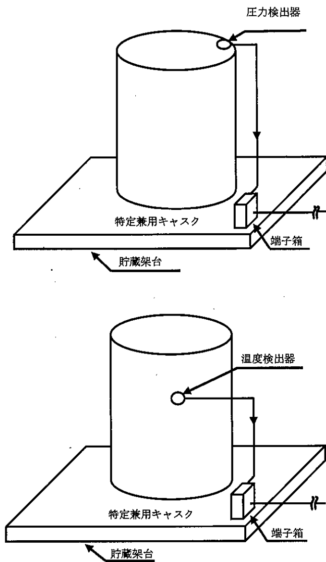
図 2.5.2-2 監視装置の構成図 (特定兼用キャスクを基礎等に固定する設置方法の例)
