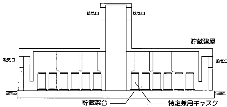
A-A矢視
