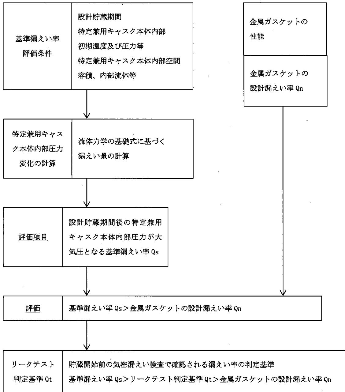
図 1-9 閉じ込め評価フロー図
