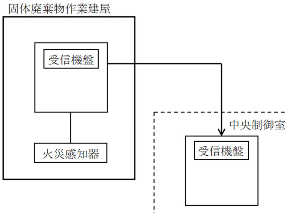
第1図 固体廃棄物作業建屋の火災感知設備の概要
