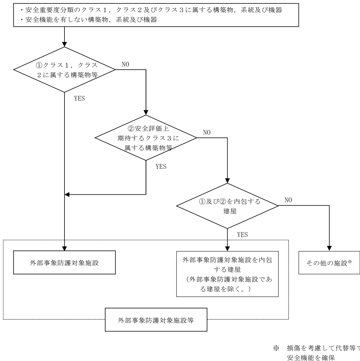
第6-1図 外部事象防護対象施設の抽出フロー
