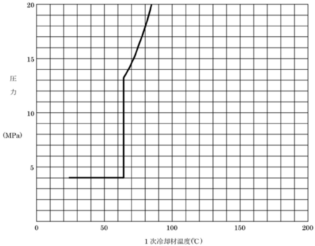
通常運転時の加熱制限曲線
