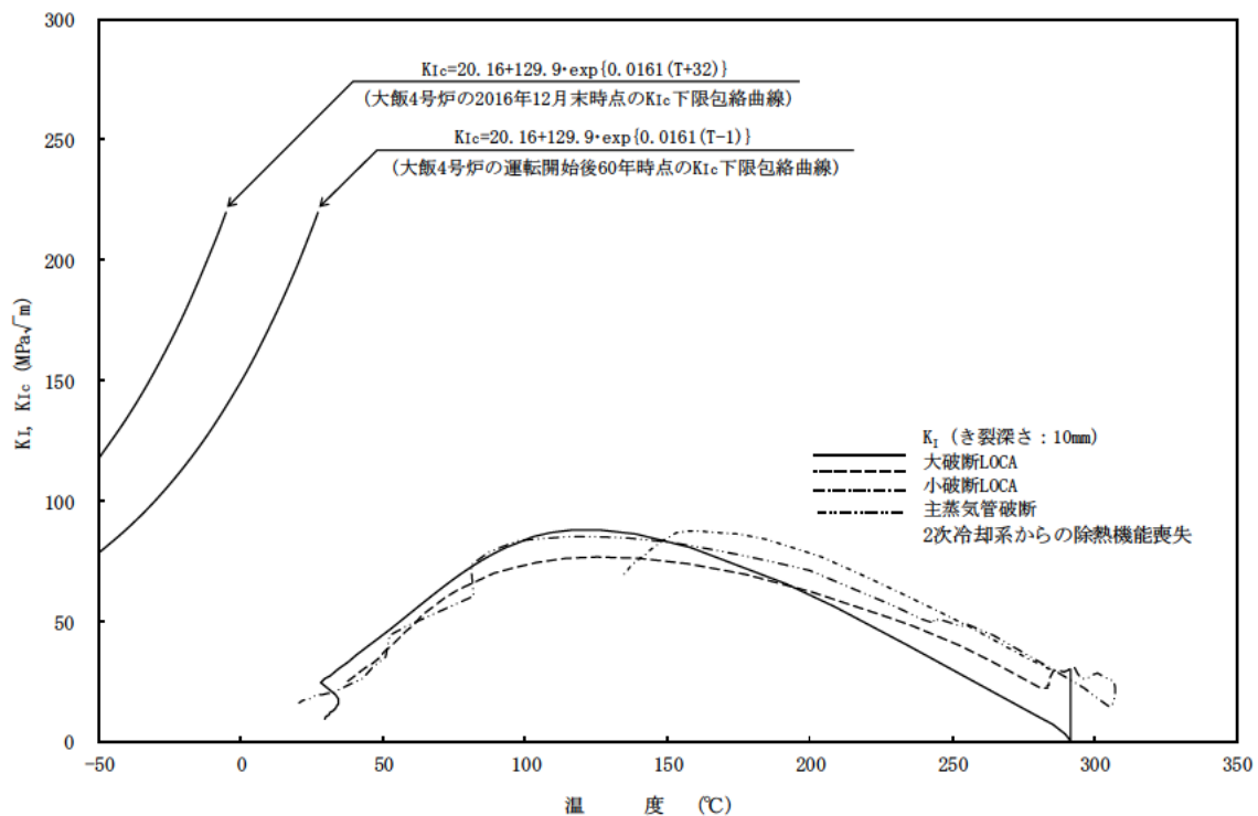
大飯4号炉 原子炉容器胴部（炉心領域部）中性子照射脆化に対するPTS評価結果 [深さ10mmの想定き裂を用いた評価]
