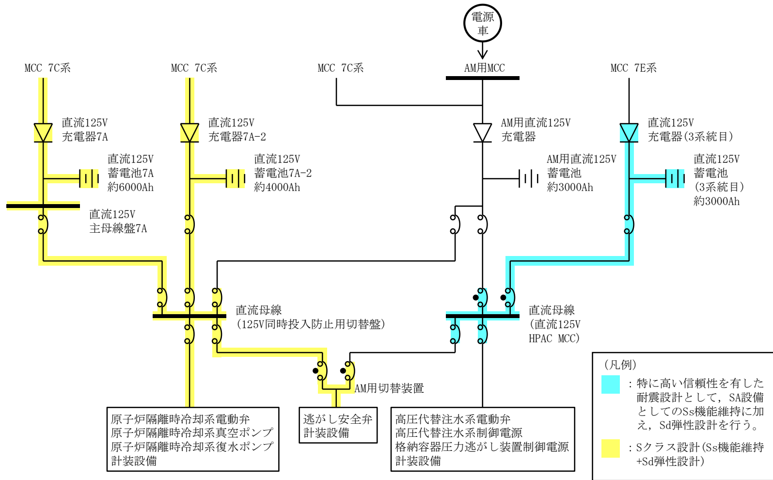
第 57-4-6 図 特に高い信頼性を有した電源設備の耐震設計範囲 (7号炉)
