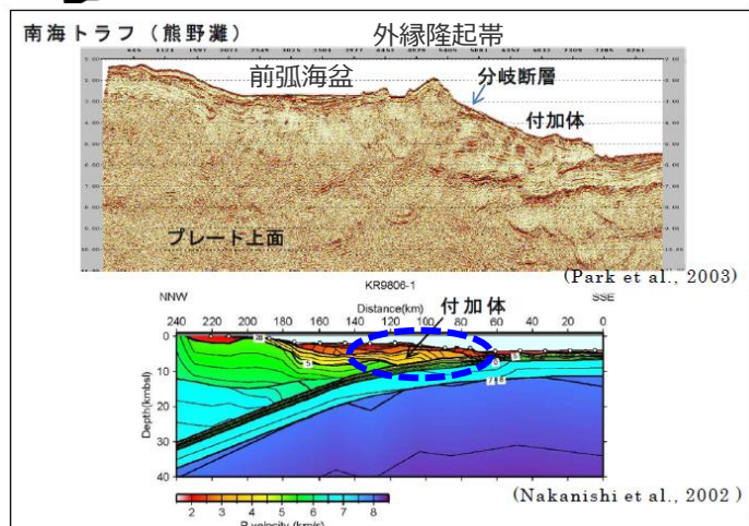
(A)南海トラフ：付加作用の卓越する沈み込み帯
