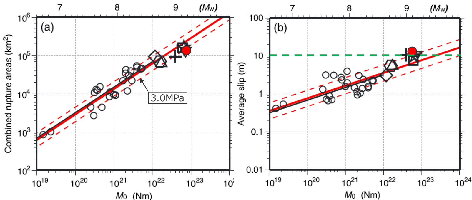
断層面積と地震モーメント
