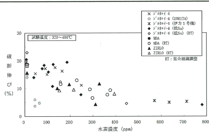
図 5-3 被覆管水素濃度と破断伸びの関係 (40)
