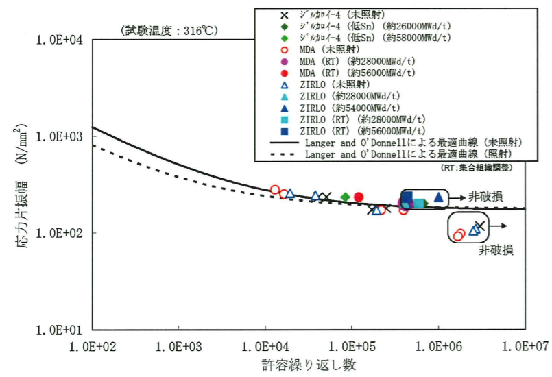
図 2.2-4 MDA及びZIRLO被覆管の疲労強度 [1, 2]
