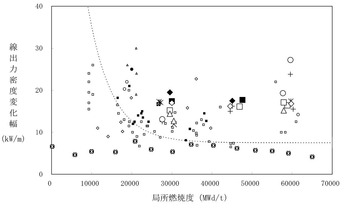
図 3-18 (1) 被覆管の出力ランプ試験結果 (6)、(13)～(15) (最大線出力密度が最大の場合の出力変化)
