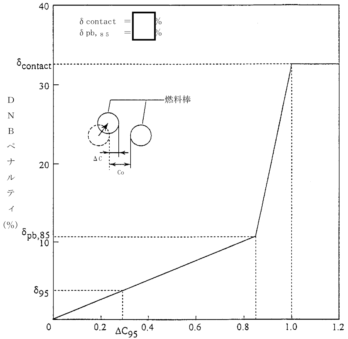
燃料棒間投影クリアランス減少量、 \Delta C/C_0
