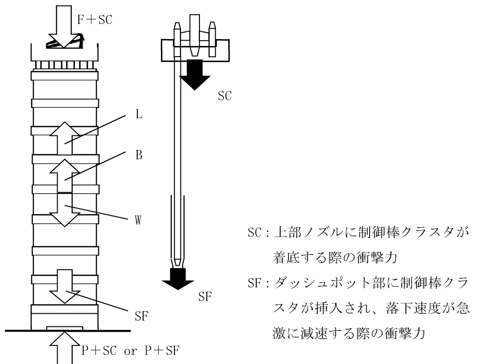
図 4-4 通常運転時及び運転時の異常な過渡変化時荷重
