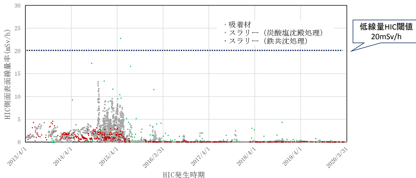
図1 一時保管施設に保管したHICの発生時期と表面線量率の分布
