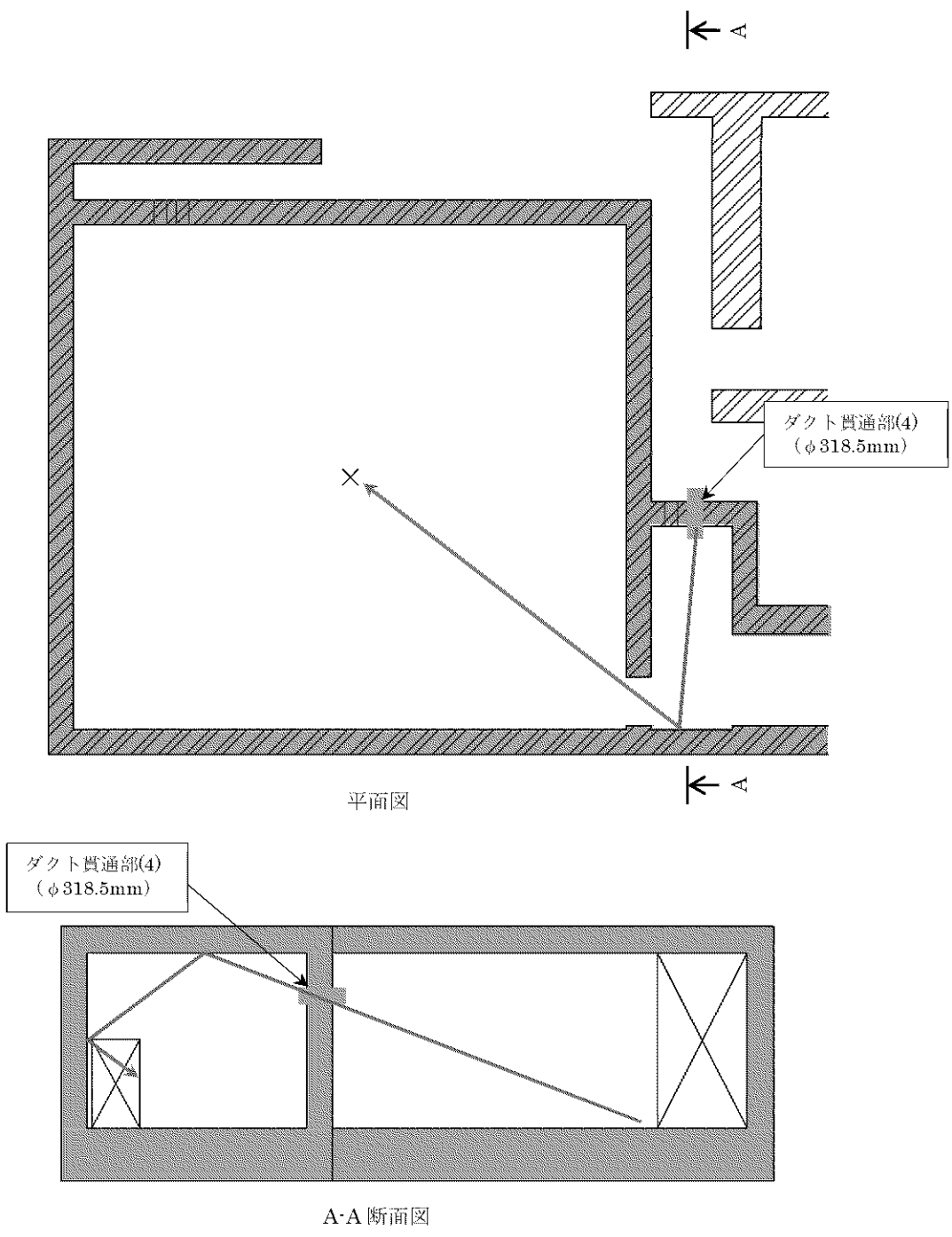
第 8 図 ダクト貫通部(4)から評価点までの散乱経路 (代表例)
