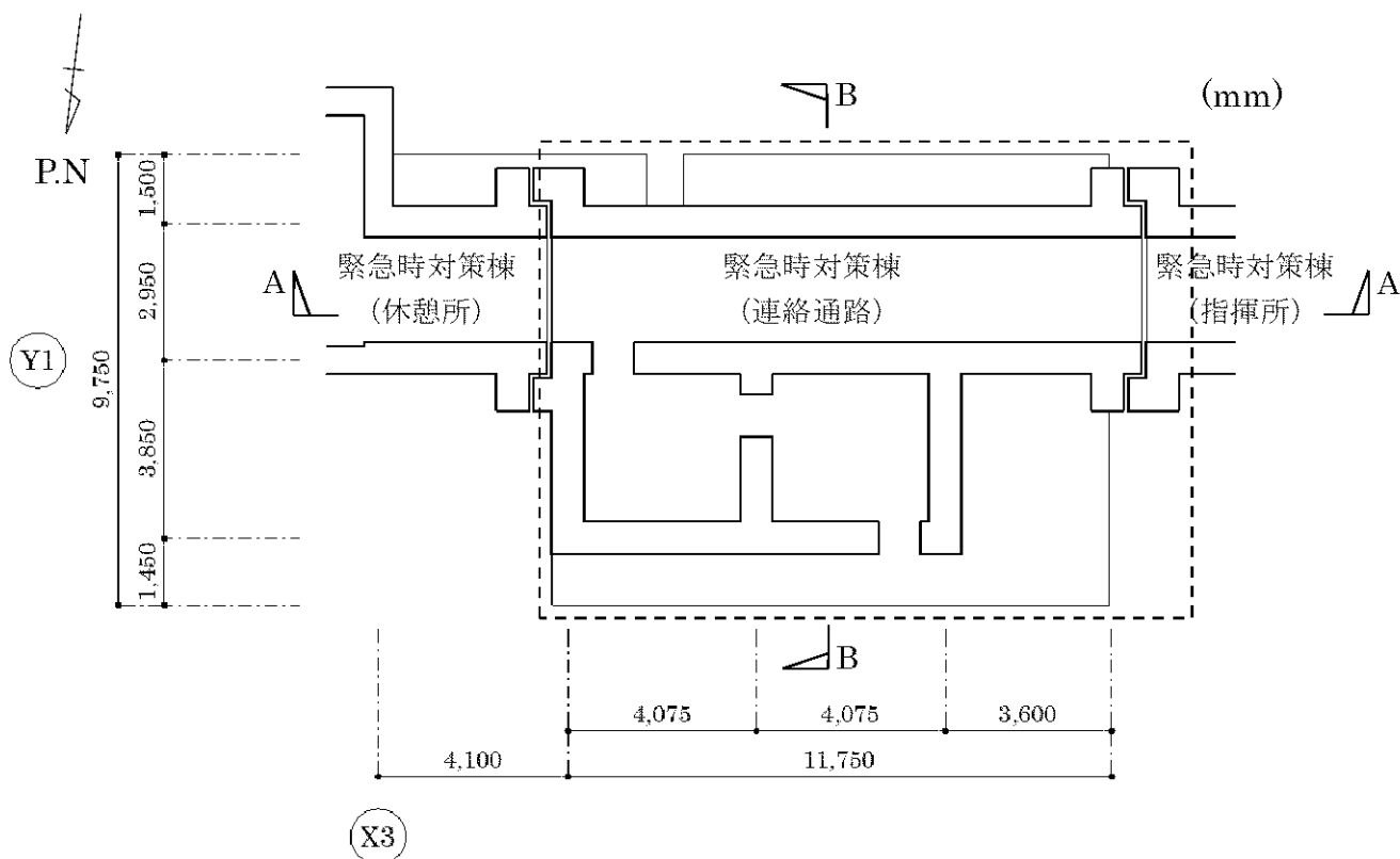
第 2-1 図 連絡通路の概略平面図
