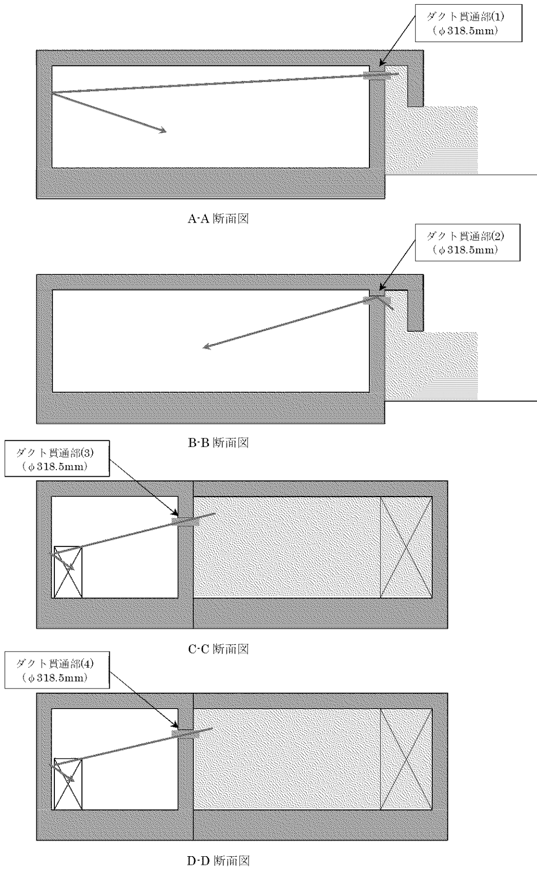
第7図 クラウド線源と評価点及び散乱経路（代表例）(2/2)
