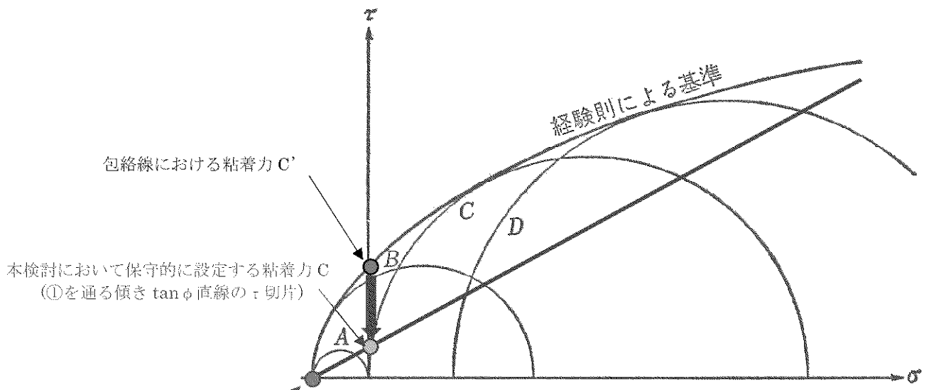
①JNES 報告書における付着力試験検を踏まえて設定する引張方向の粘着力 図 3.19 モールの円に包絡線を描いて作成した実験結果による破壊基準：A, 引張り：B, 圧裂：C, 一軸圧縮：D, 三軸圧縮
