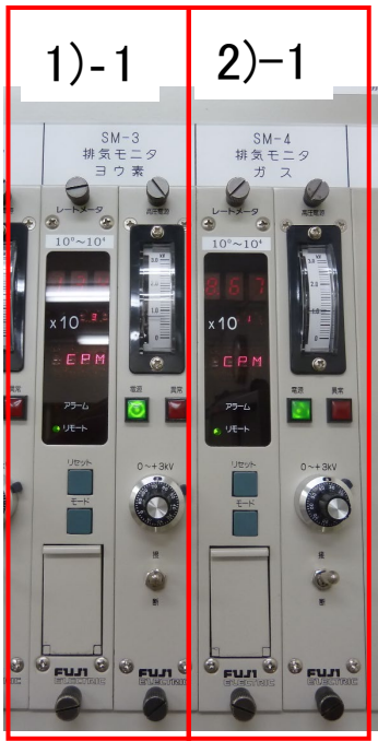
1)-1 ヨウ素モニタ指示計 2)-1 ガスモニタ指示計
