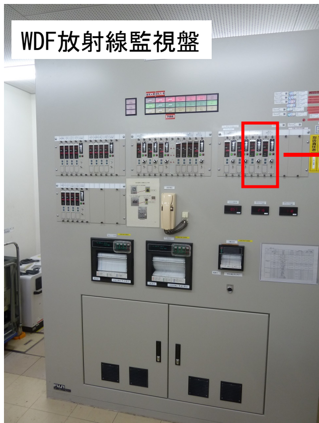
1)-1 ヨウ素モニタ指示計 2)-1 ガスモニタ指示計
