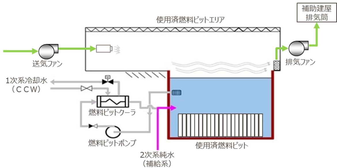
図2 試験時の概略系統
