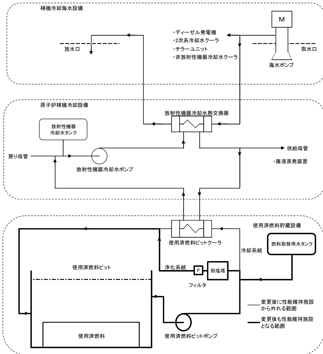
図 12 使用済燃料の貯蔵に係る性能維持施設の範囲 (変更後)
