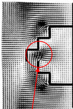
渦動粘性係数 100m 2 /s
