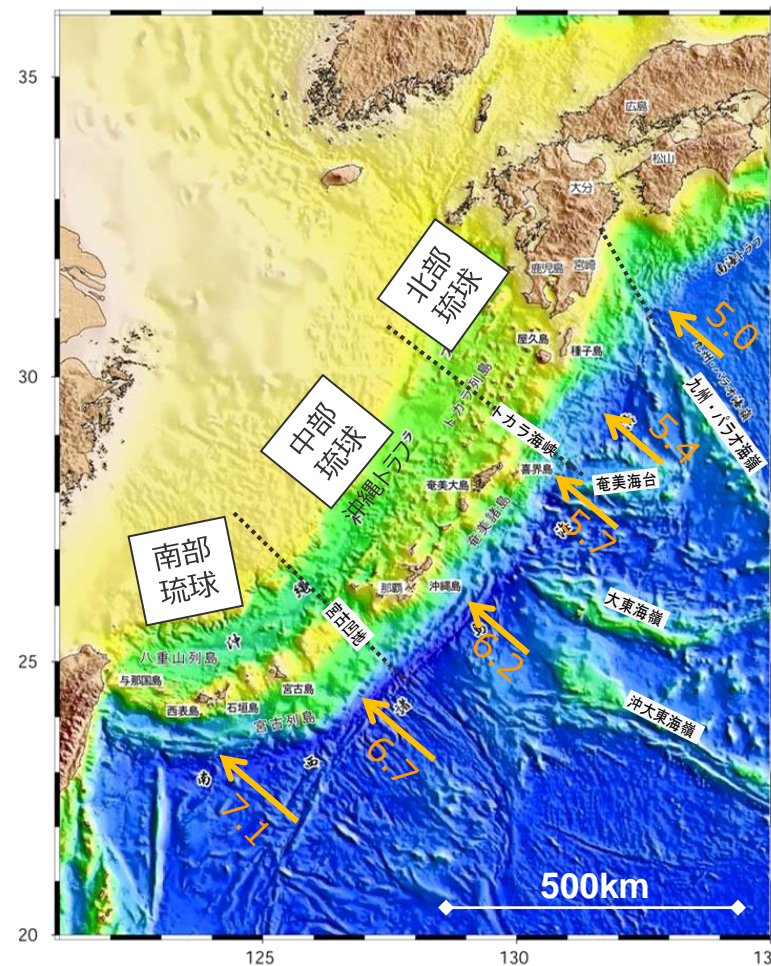
(地震調査委員会(2004a)、Seno et al.(1993)に基づき作成)
