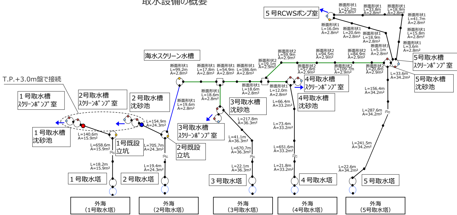
取水設備の解析モデル※2
