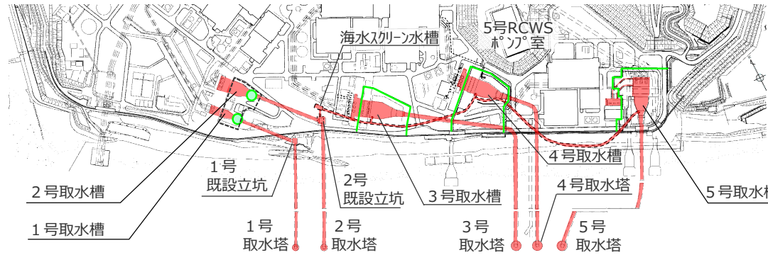
取水設備の概要
