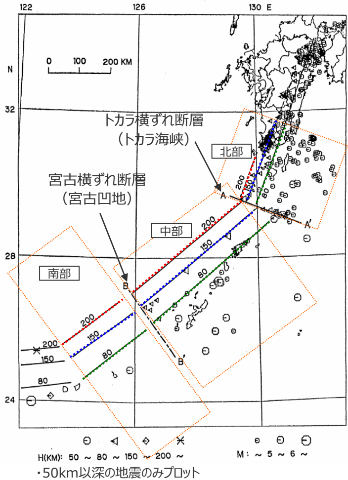
琉球海溝のスラブの傾斜（長宗(1987)に加筆）
