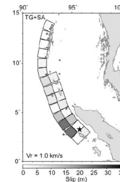
ライズタイム：180s （すべり速度：0.1m/s）
