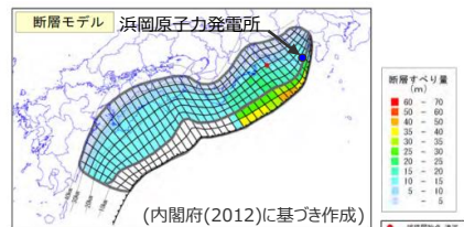
【基本的な検討ケース】ケース①
