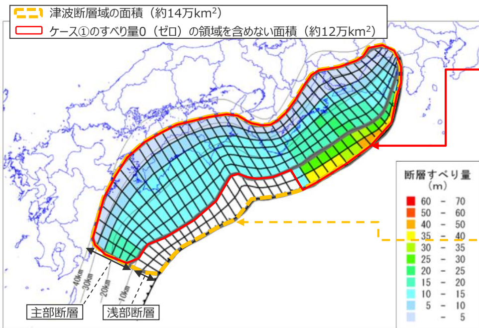
内閣府の最大クラスモデル（ケース①の例）
