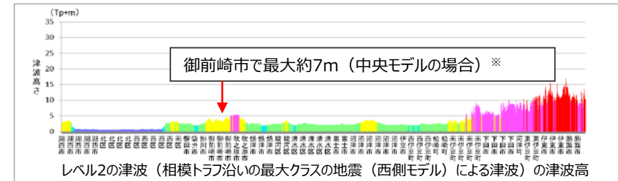
レベル2の津波(相模トラフ沿いの最大クラスの地震(西側モデル)による津波)の津波高 * 静岡県(2015)に西側モデルの図のみ記載。御前崎市での最大は中央モデルであることから併記 (静岡県(2015)に基づき作成)
