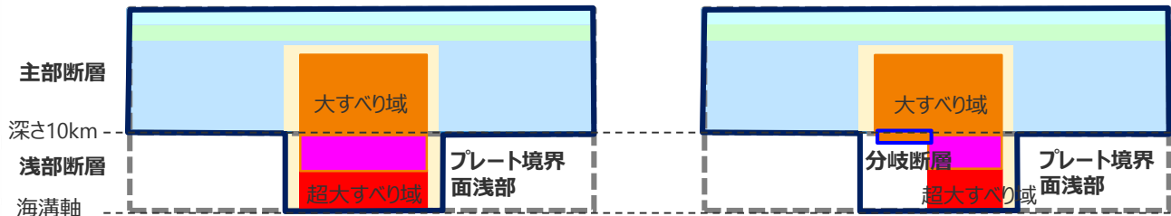
内閣府の最大クラスモデルのすべり量分布概念図
