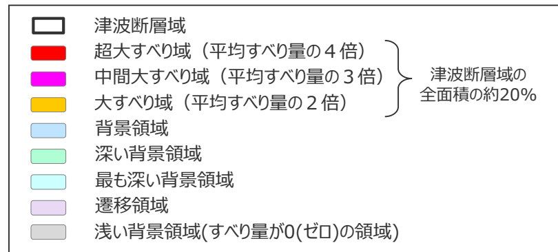
パラメータスタディモデルの小断層のすべり量分布 (m)
