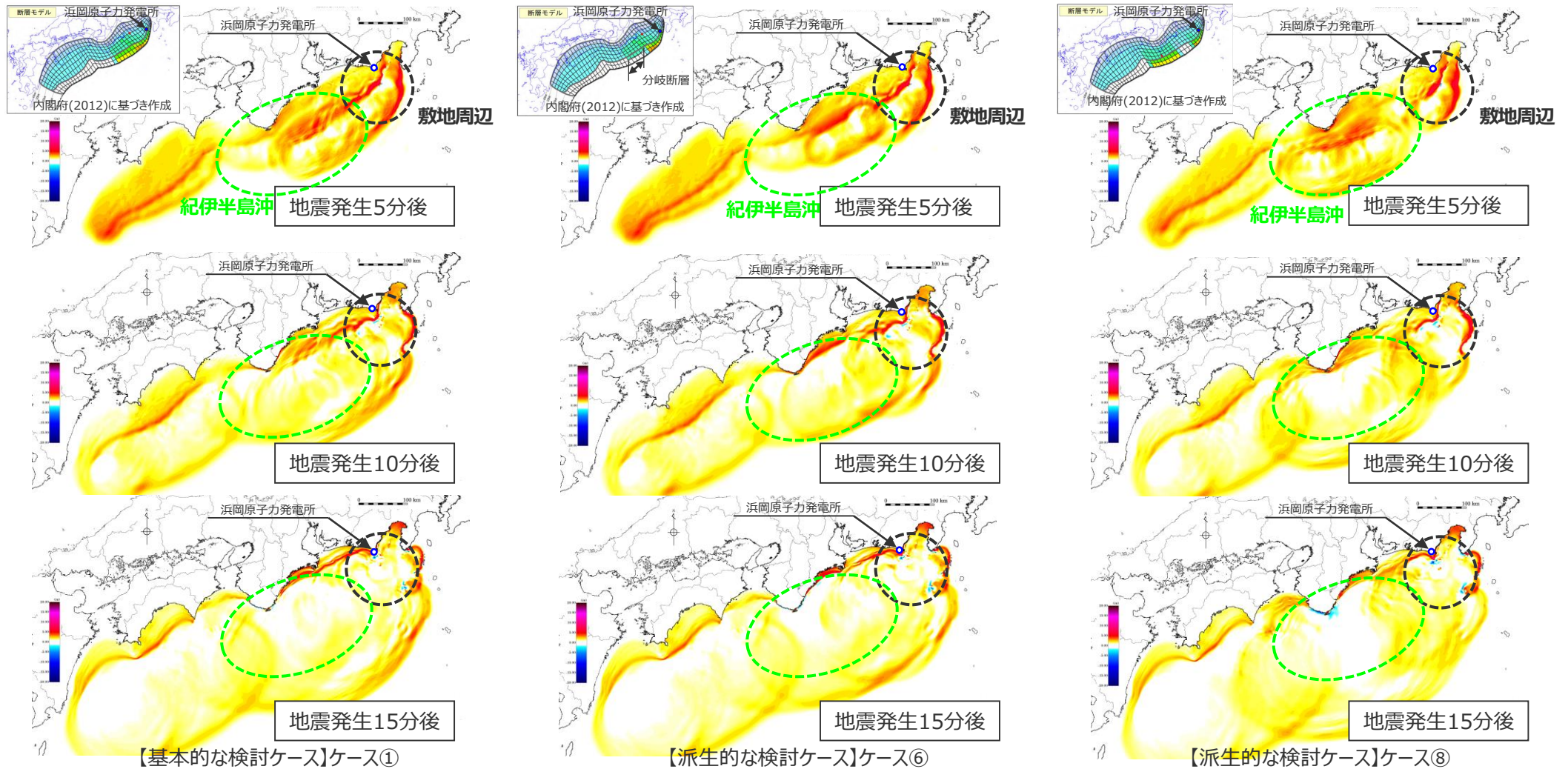
内閣府の最大クラスモデルの津波伝播状況スナップショット
