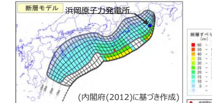
【派生的な検討ケース】ケース⑧
