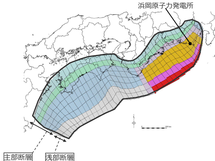
パラメータスタディモデル
