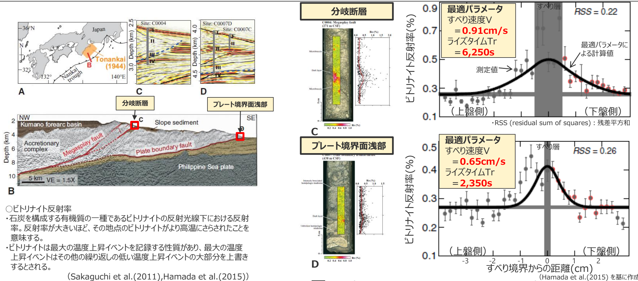
ビトリナイト反射率 (Ro) 分布の測定値とライズタイム等の算定
