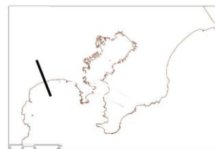
国府津-松田断層帯の波源モデル
