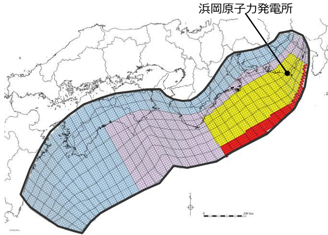
日本海溝の特性化手法モデル② （日本海溝の特性化手法②）
