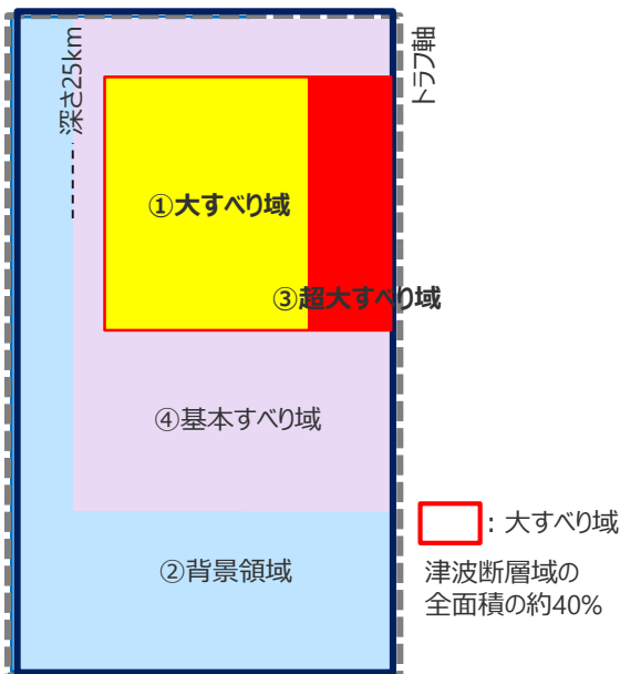
日本海溝の特性化手法モデル②による すべり量分布概念図
