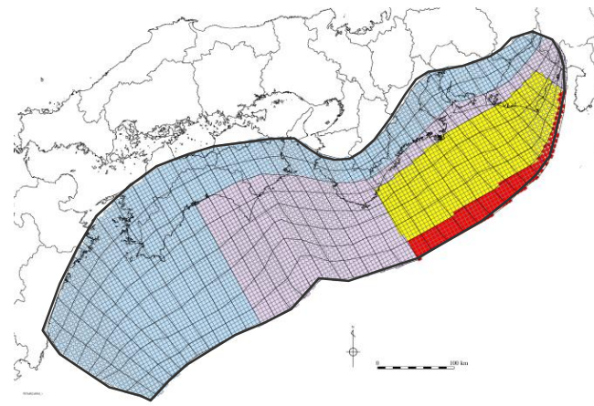
日本海溝の特性化手法モデル②
