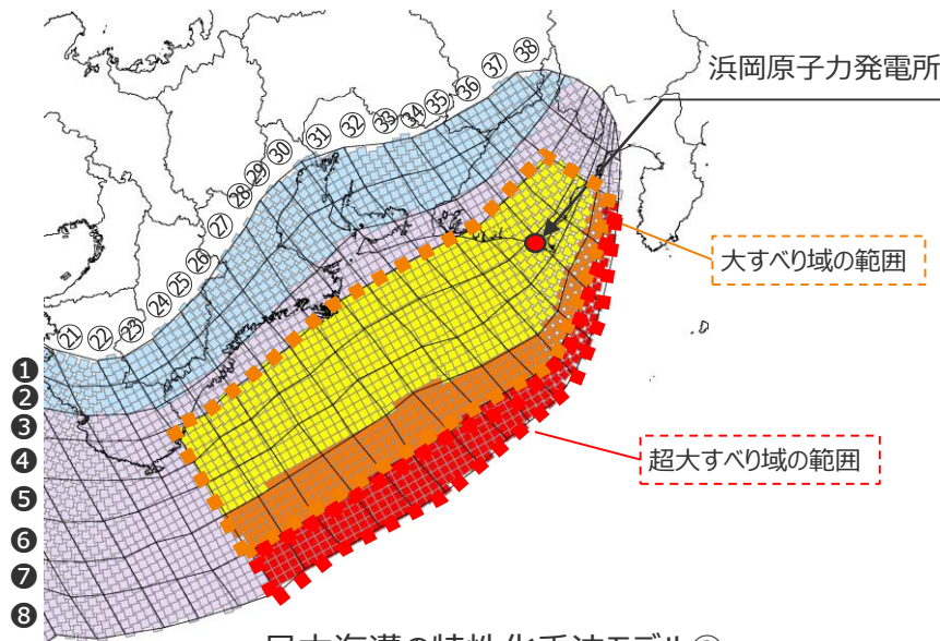
日本海溝の特性化手法モデル③
