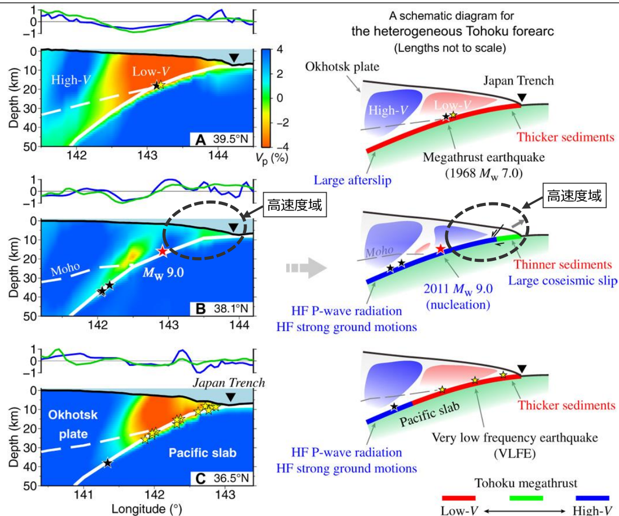
2011年東北沖地震の速度分布とそのイメージ (Liu and Zhao(2018)を基に作成)
