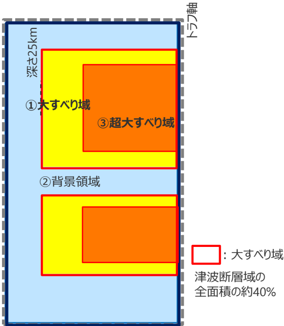
日本海溝の特性化手法モデル①によるすべり量分布概念図
