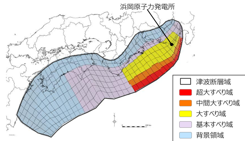
日本海溝の特性化手法モデル③（日本海溝の特性化手法③）
