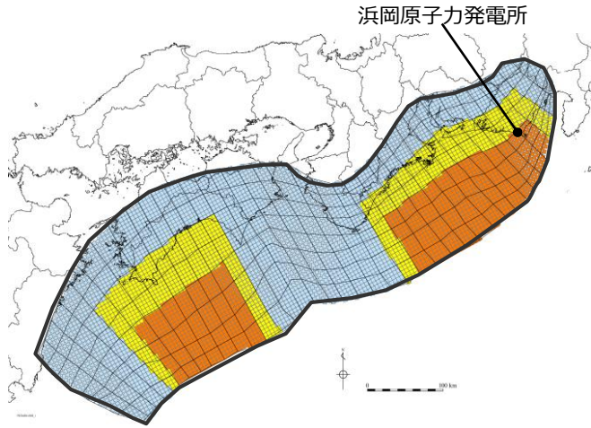
日本海溝の特性化手法モデル① （日本海溝の特性化手法①）
