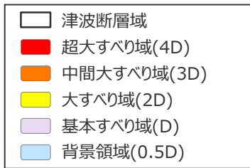
日本海溝の特性化手法モデル③
