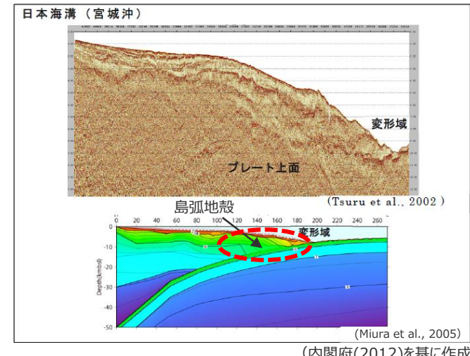
(B)東北沖：造構性侵食作用が卓越する沈み込み帯
