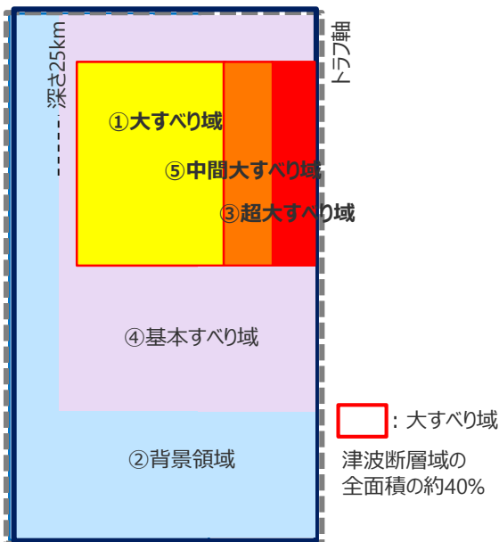
日本海溝の特性化手法モデル③による すべり量分布概念図
