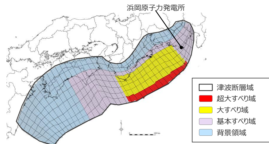
日本海溝の特性化手法モデル② の大すべり域の位置を西へ70kmとしたケース
