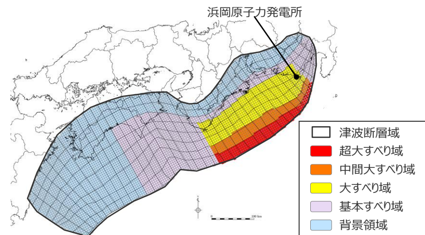
日本海溝の特性化手法モデル③ の大すべり域の位置を西へ30kmとしたケース
