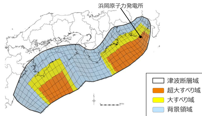
日本海溝の特性化手法モデル① の大すべり域の位置を東へ10kmとしたケース
