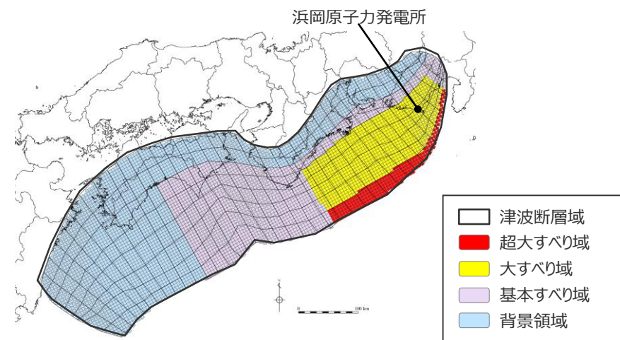
日本海溝の特性化手法モデル② の大すべり域の位置を東へ10kmとしたケース
