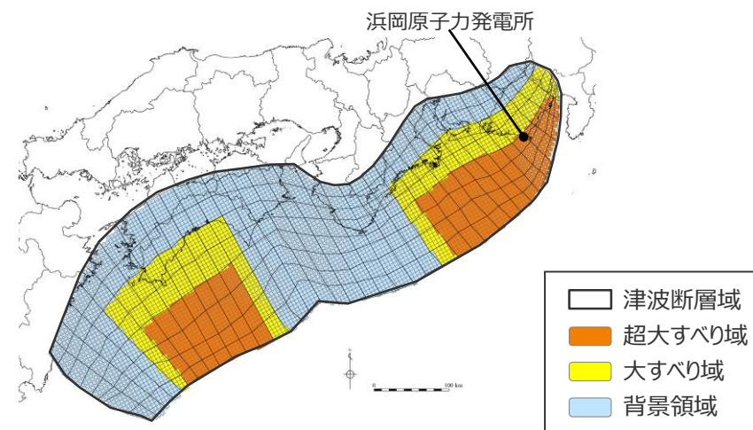
日本海溝の特性化手法モデル① の大すべり域の位置を東へ40kmとしたケース
