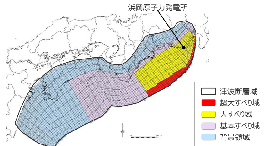
日本海溝の特性化手法モデル② の大すべり域の位置を東へ20kmとしたケース
