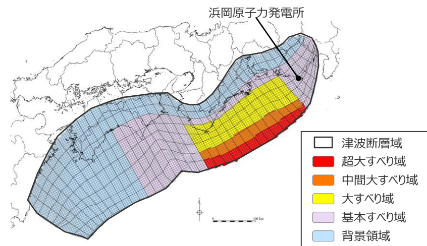
日本海溝の特性化手法モデル③ の大すべり域の位置を西へ80kmとしたケース
