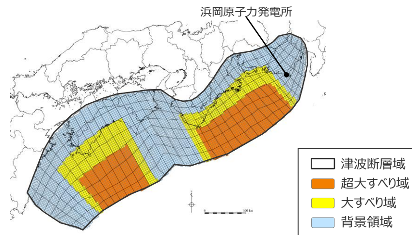
日本海溝の特性化手法モデル① の大すべり域の位置を西へ70kmとしたケース
