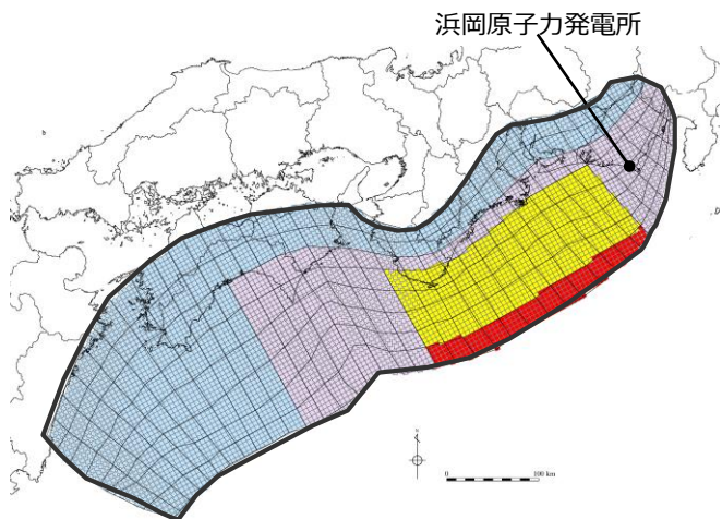
日本海溝の特性化手法モデル②の大すべり域の位置を西へ80kmとしたケース
