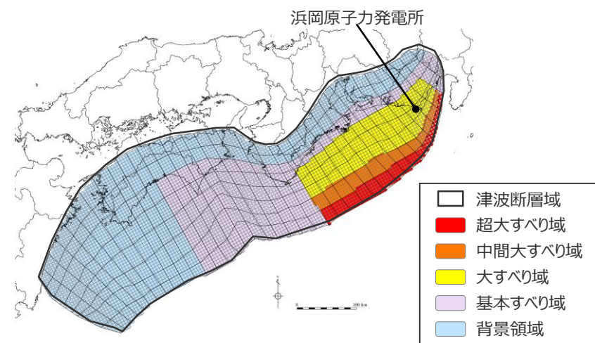
日本海溝の特性化手法モデル③ の大すべり域の位置を基準位置としたケース
