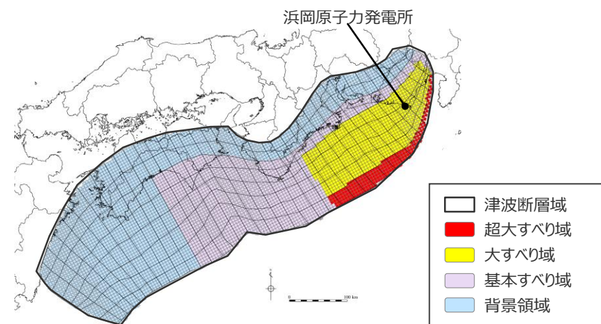
日本海溝の特性化手法モデル② の大すべり域の位置を東へ30kmとしたケース
