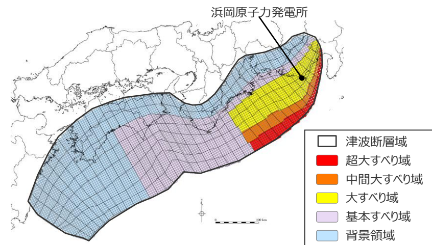
日本海溝の特性化手法モデル③ の大すべり域の位置を東へ40kmとしたケース
