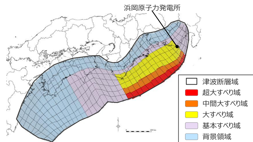
日本海溝の特性化手法モデル③ の大すべり域の位置を西へ40kmとしたケース
