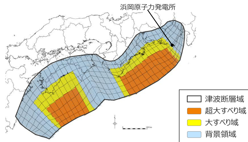
日本海溝の特性化手法モデル① の大すべり域の位置を西へ50kmとしたケース
