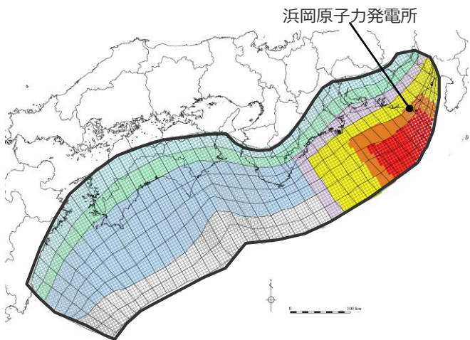
検討波源モデルDの大すべり域の位置を東へ50kmとしたケース
