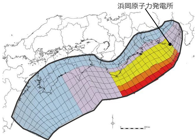
日本海溝の特性化手法モデル③の大すべり域の位置を西へ40kmとしたケース
