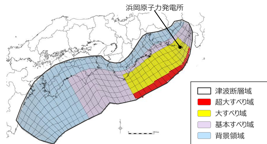
日本海溝の特性化手法モデル② の大すべり域の位置を西へ20kmとしたケース
