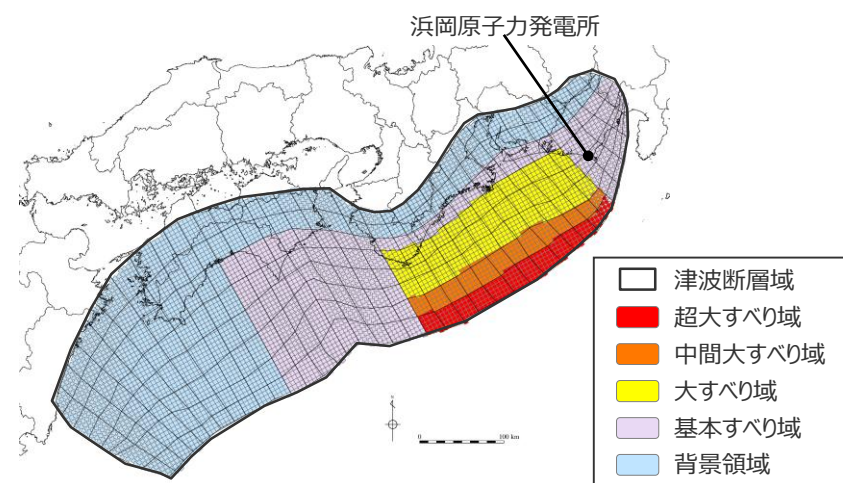
日本海溝の特性化手法モデル③ の大すべり域の位置を西へ60kmとしたケース
