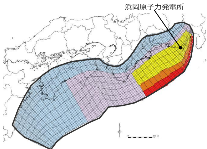
日本海溝の特性化手法モデル③の大すべり域の位置を東へ20kmとしたケース
