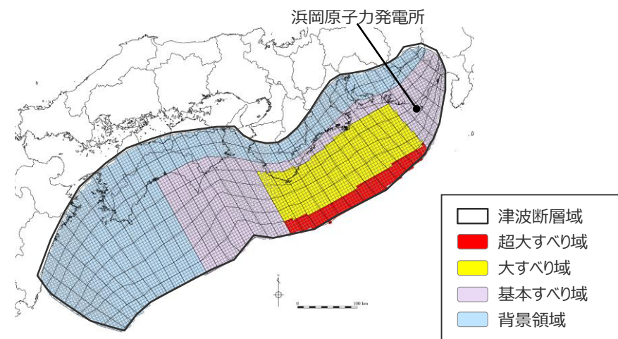
日本海溝の特性化手法モデル② の大すべり域の位置を西へ80kmとしたケース
