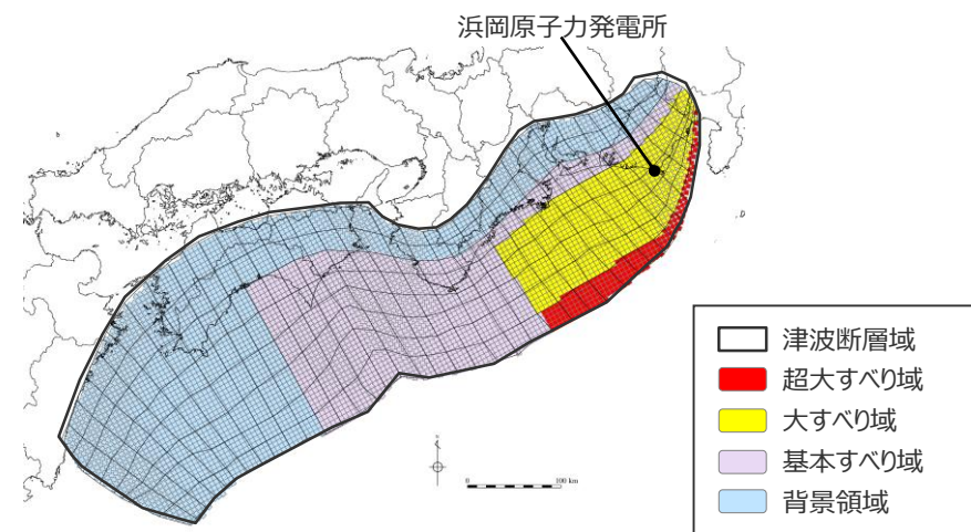
日本海溝の特性化手法モデル② の大すべり域の位置を東へ40kmとしたケース
