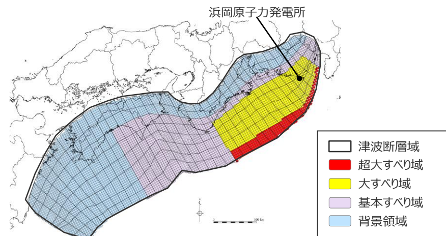
日本海溝の特性化手法モデル② の大すべり域の位置を基準位置としたケース
