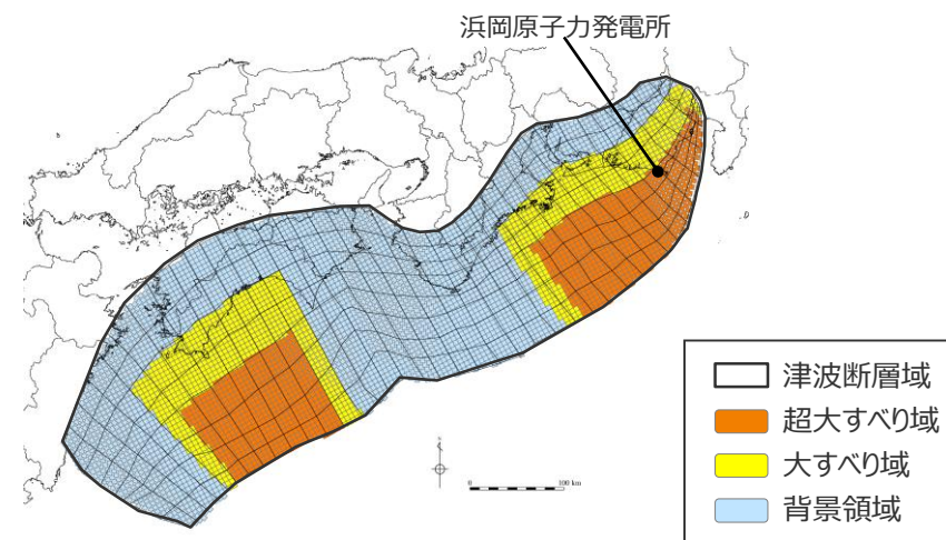
日本海溝の特性化手法モデル① の大すべり域の位置を東へ50kmとしたケース
