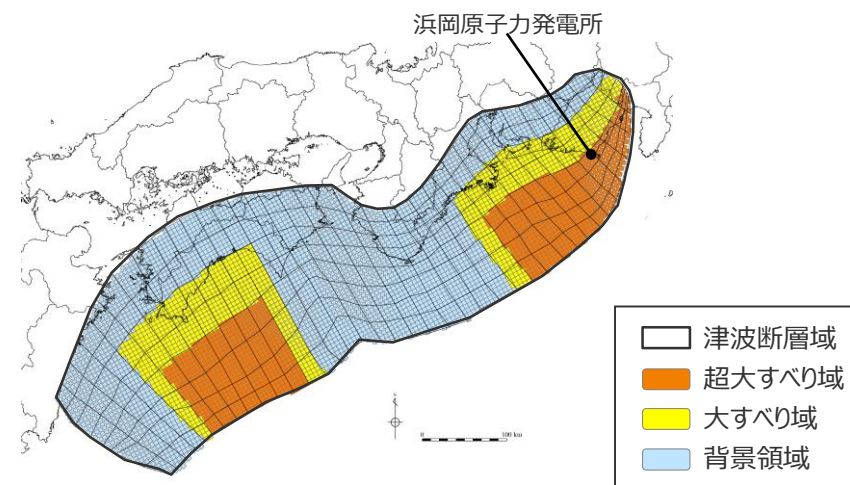
日本海溝の特性化手法モデル① の大すべり域の位置を東へ60kmとしたケース
