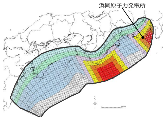
検討波源モデルDの敷地に近い大すべり域の位置を東へ40km、大すべり域間の距離を80kmとしたケース
