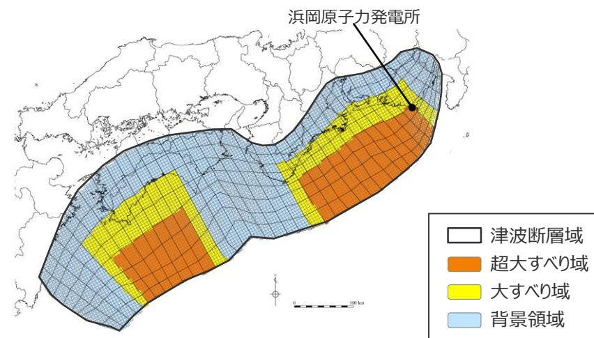
日本海溝の特性化手法モデル① の大すべり域の位置を西へ20kmとしたケース
