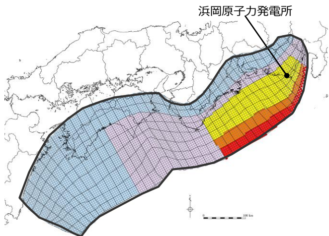
日本海溝の特性化手法モデル③の大すべり域の位置を基準位置としたケース
