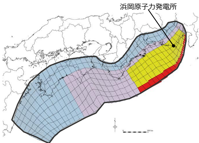
日本海溝の特性化手法モデル②の大すべり域の位置を東へ20kmとしたケース
