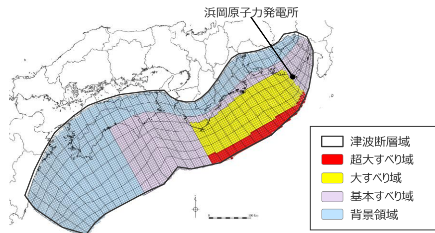
日本海溝の特性化手法モデル② の大すべり域の位置を西へ50kmとしたケース
