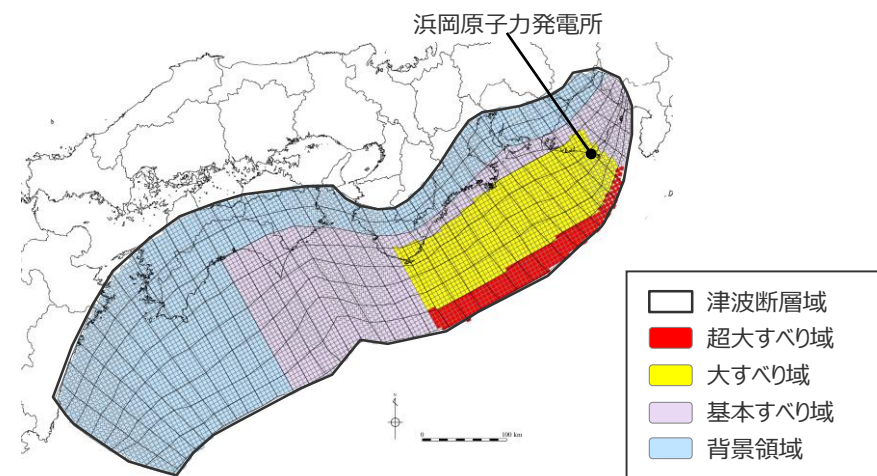
日本海溝の特性化手法モデル② の大すべり域の位置を西へ30kmとしたケース
