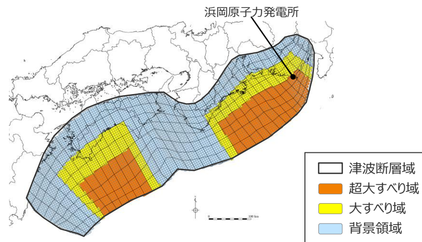
日本海溝の特性化手法モデル① の大すべり域の位置を基準位置としたケース
