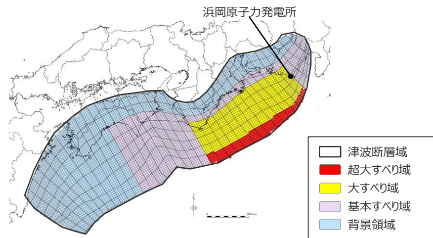
日本海溝の特性化手法モデル② の大すべり域の位置を西へ40kmとしたケース
