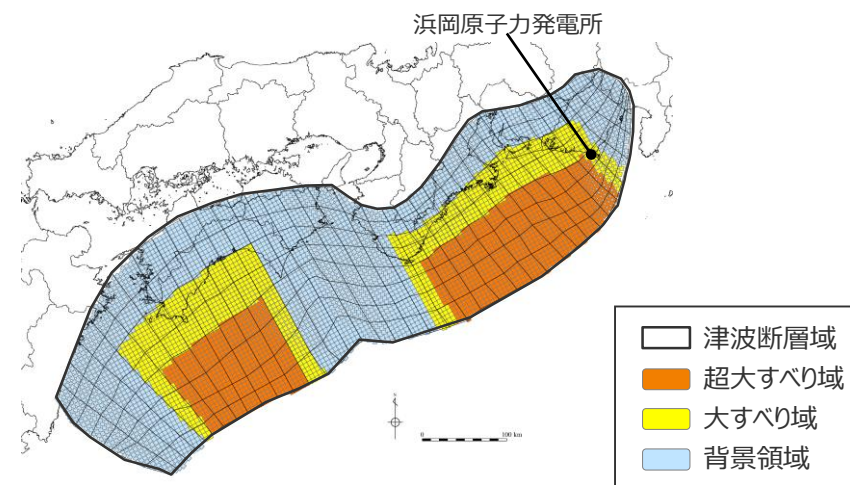
日本海溝の特性化手法モデル① の大すべり域の位置を西へ30kmとしたケース
