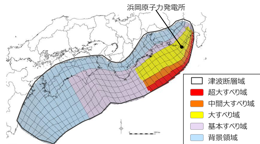
日本海溝の特性化手法モデル③ の大すべり域の位置を東へ30kmとしたケース
