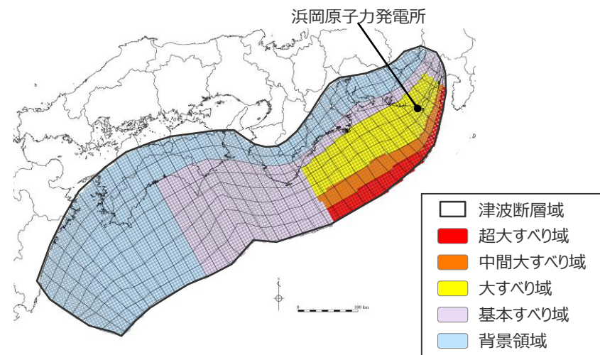
日本海溝の特性化手法モデル③ の大すべり域の位置を東へ10kmとしたケース
