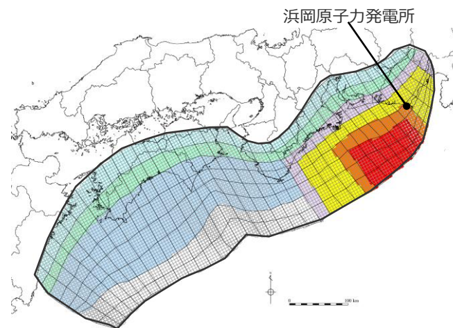
検討波源モデルD の大すべり域の位置を東へ20kmとしたケース
