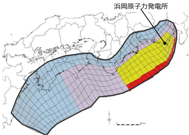
日本海溝の特性化手法モデル②の大すべり域の位置を基準位置としたケース
