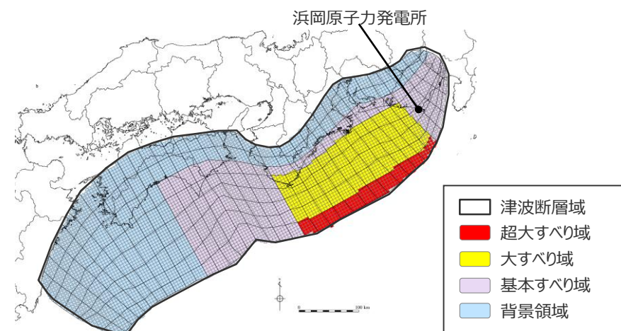
日本海溝の特性化手法モデル② の大すべり域の位置を西へ60kmとしたケース
