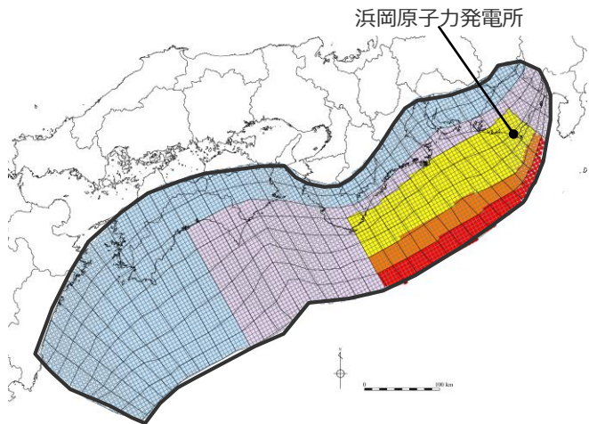
日本海溝の特性化手法モデル③の大すべり域の位置を西へ20kmとしたケース
