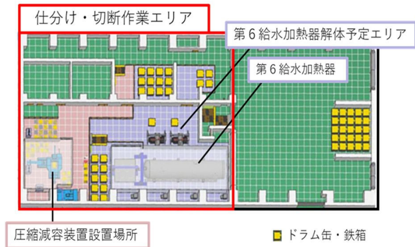
第27-2図 第6給水加熱器解体時の固体廃棄物作業建屋1階イメージ図
