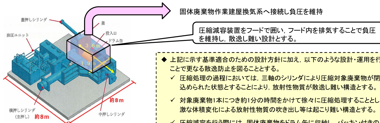
第27-3図 圧縮減容装置イメージ図 (設計進捗によりフード範囲や排気方法は変更となる可能性あり)
