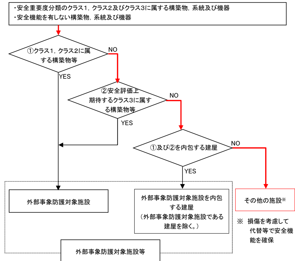
外部事象防護対象施設の抽出フロー
