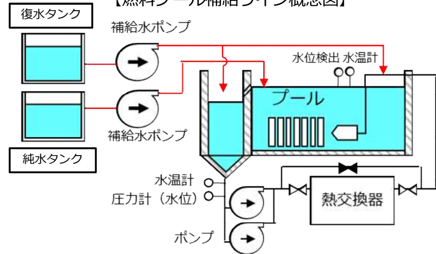
【燃料プール補給ライン概念図】
