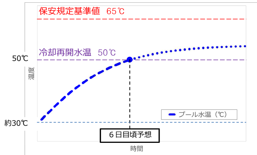
【冷却停止時のプール水温イメージ】
