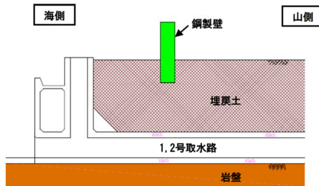
1,2号取水路断面図（水路縦断方向断面）
