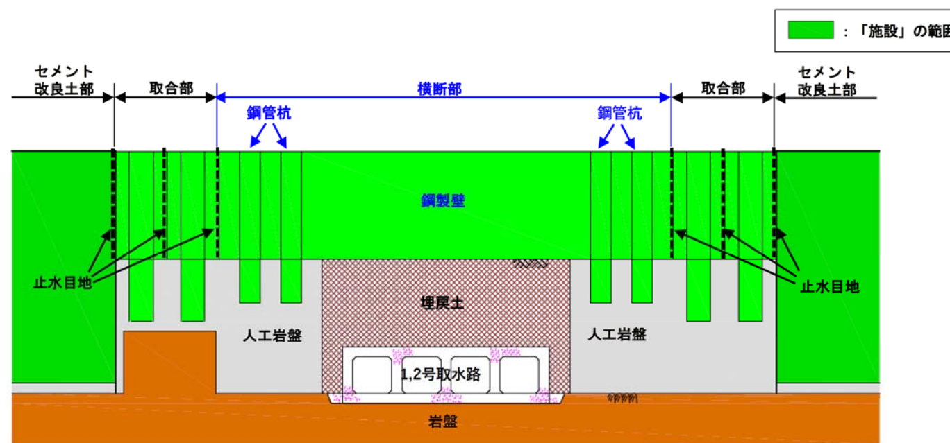
鋼製壁部(横断部)正面図
