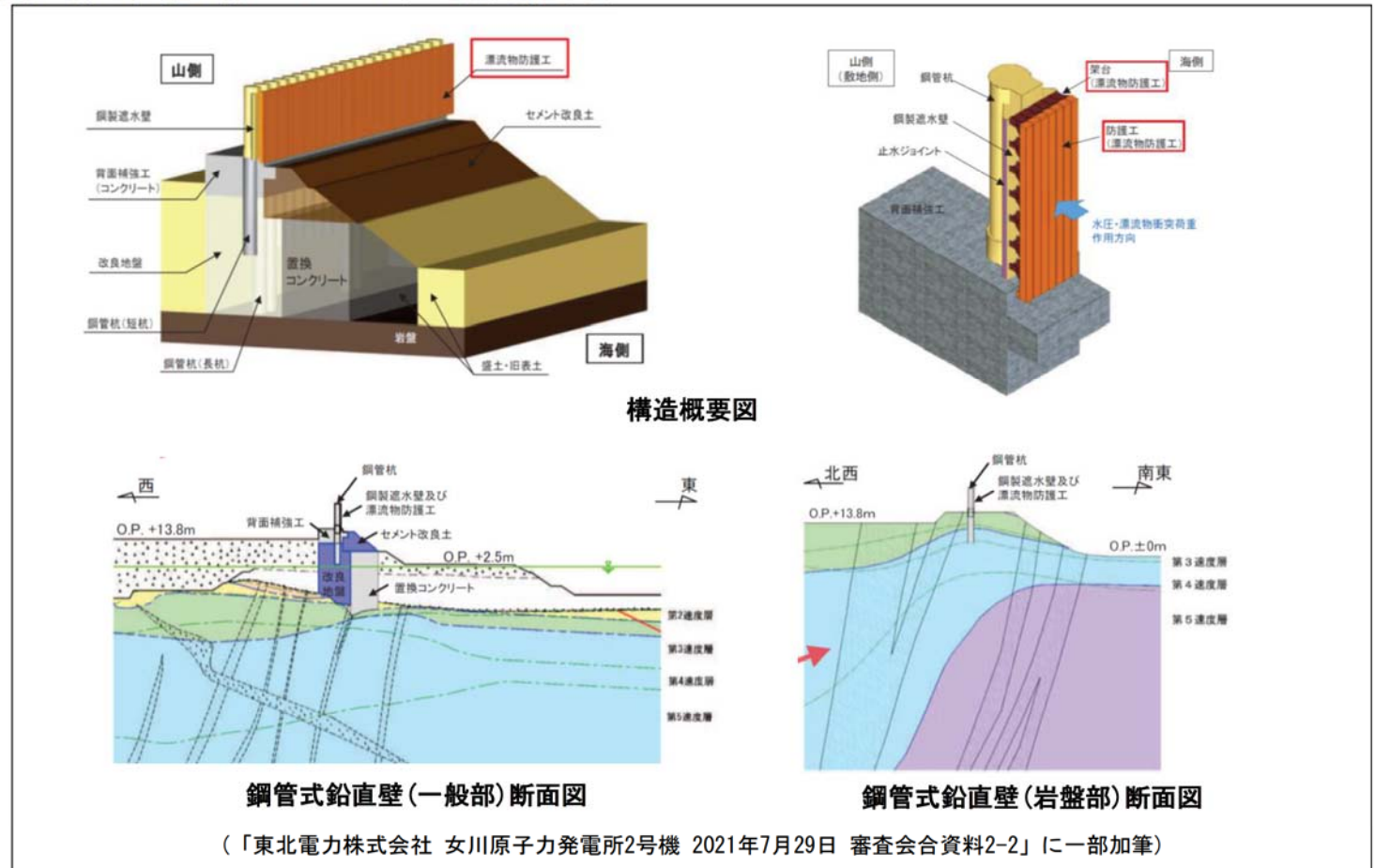
女川発電所 鋼管杭式鉛直壁
