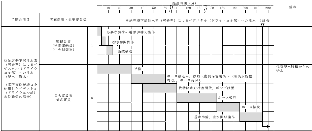
【ホース敷設 (代替淡水貯槽から高所東側接続口) の場合は 402m】
