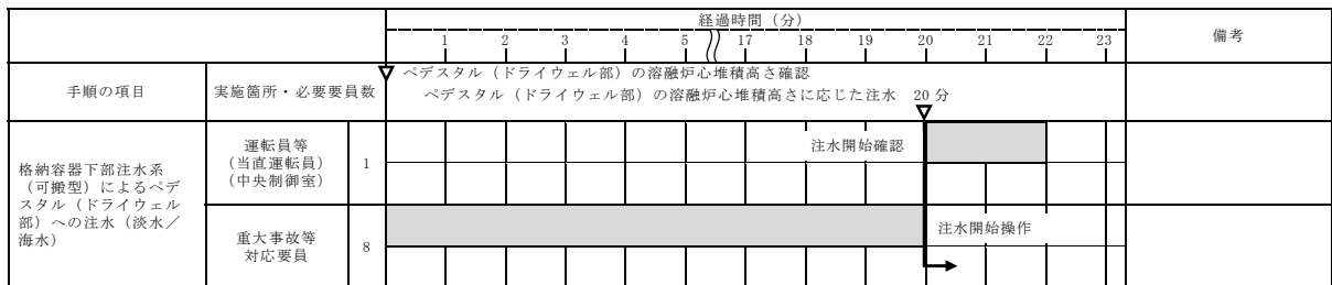
【原子炉圧力容器破損後のペDESTAL (ドライウエル部) への注水】
