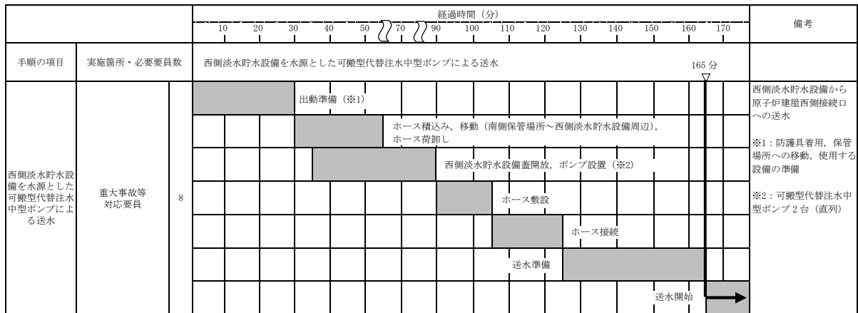
【ホース敷設にホース運搬車を使用する場合, 原子炉建屋西側接続口への送水開始まで 160 分以内で可能である。】
