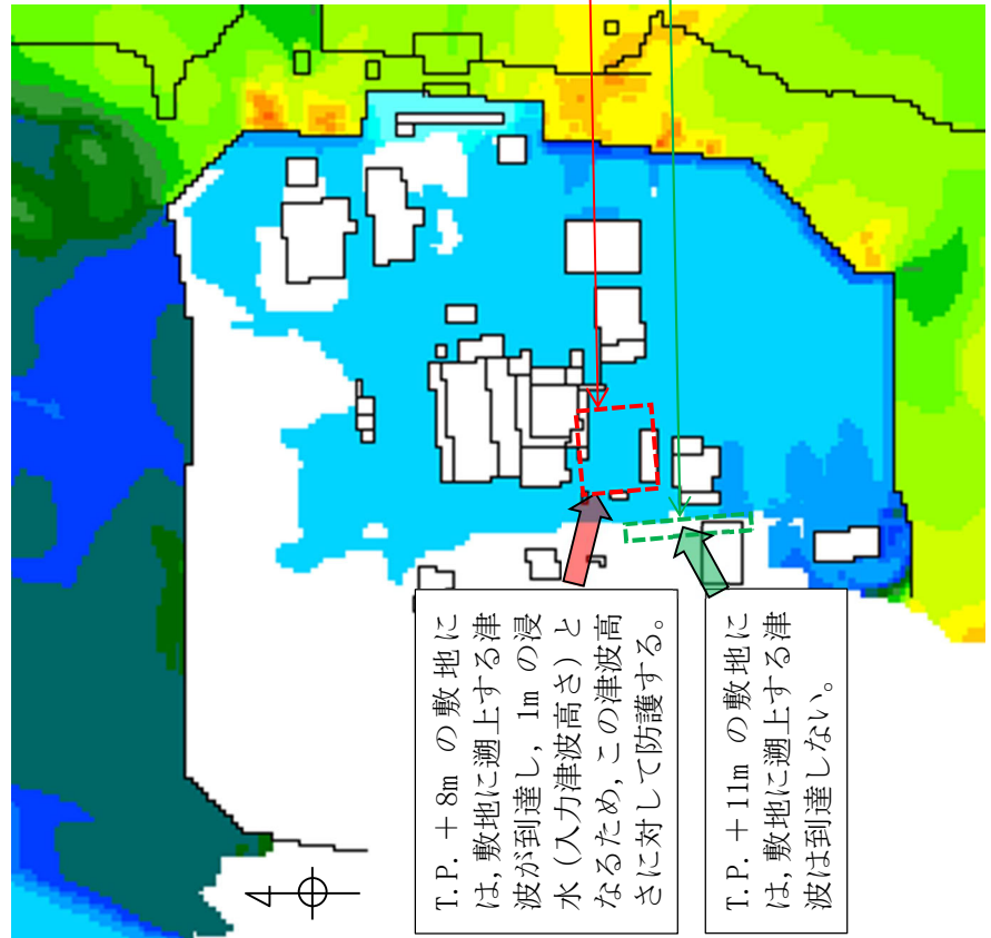
(a) 敷地に遡上する津波が流入する範囲
