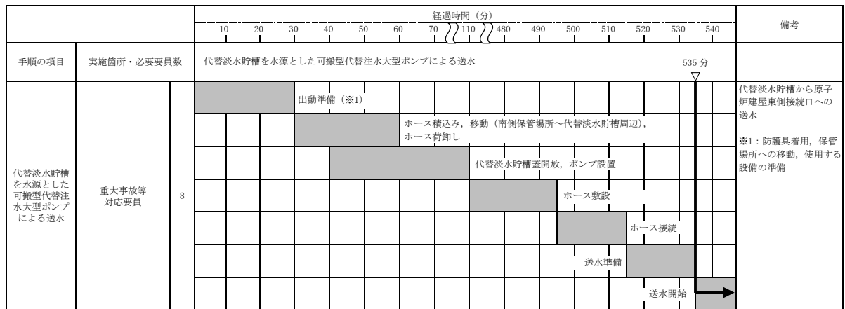
【ホース敷設にホース運搬車を使用する場合, 原子炉建屋東側接続口への送水開始まで 205 分以内で可能である。】
