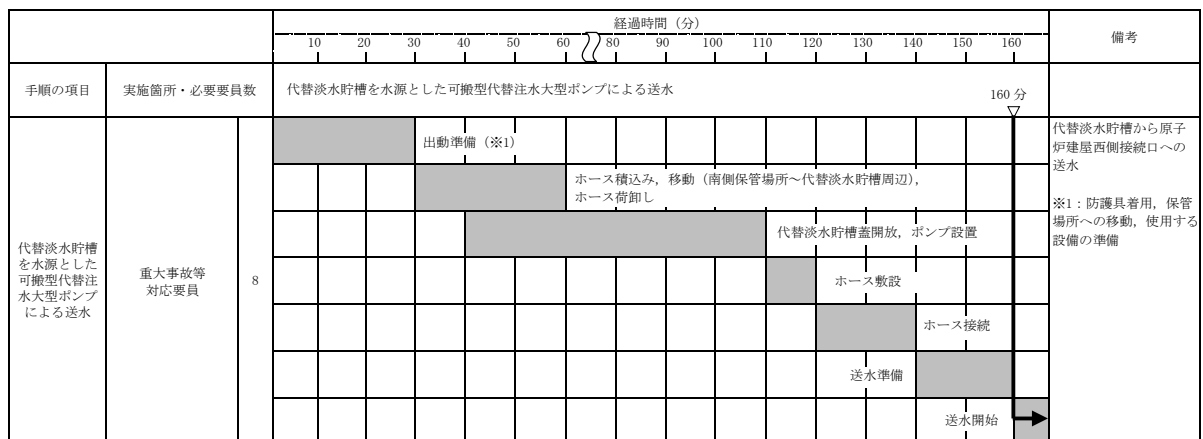
【ホース敷設にホース運搬車を使用する場合, 原子炉建屋西側接続口への送水開始まで 145 分以内で可能である。】
