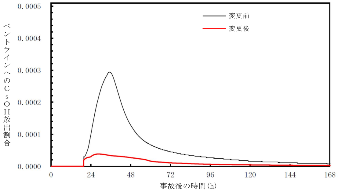
第3図 ベントラインへのCsOH放出割合 * の推移 (瞬時値)
