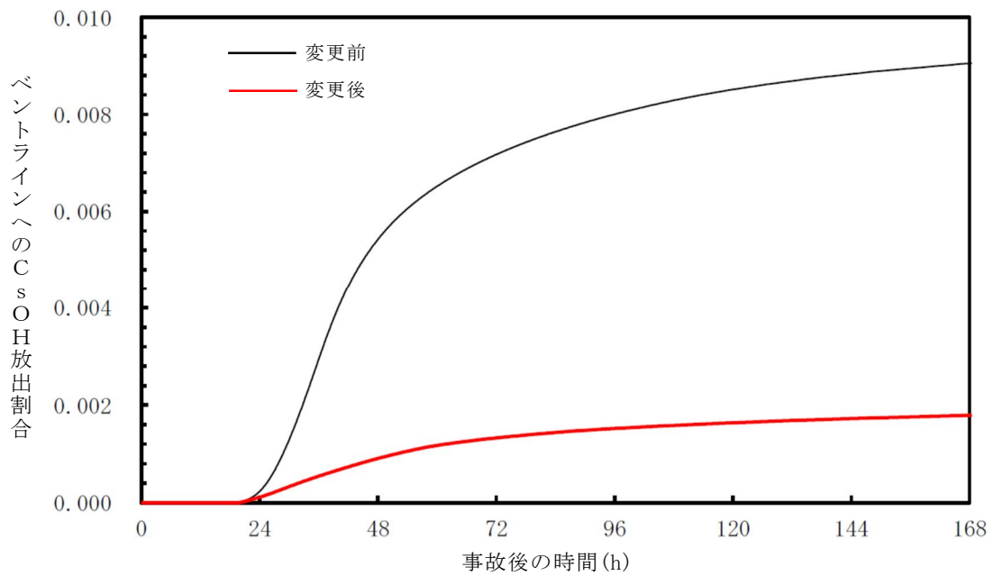
第3図 ベントラインへのCsOH放出割合 ※ の推移（積算値）
