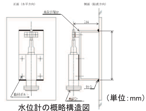
水位計の概略構造図
