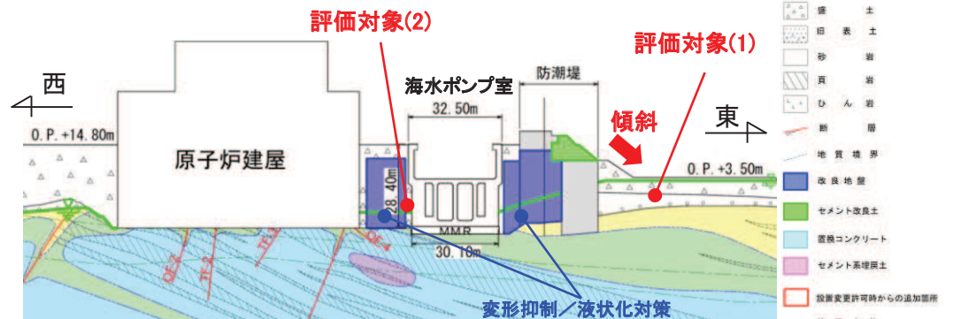
横断面(B-B断面)
