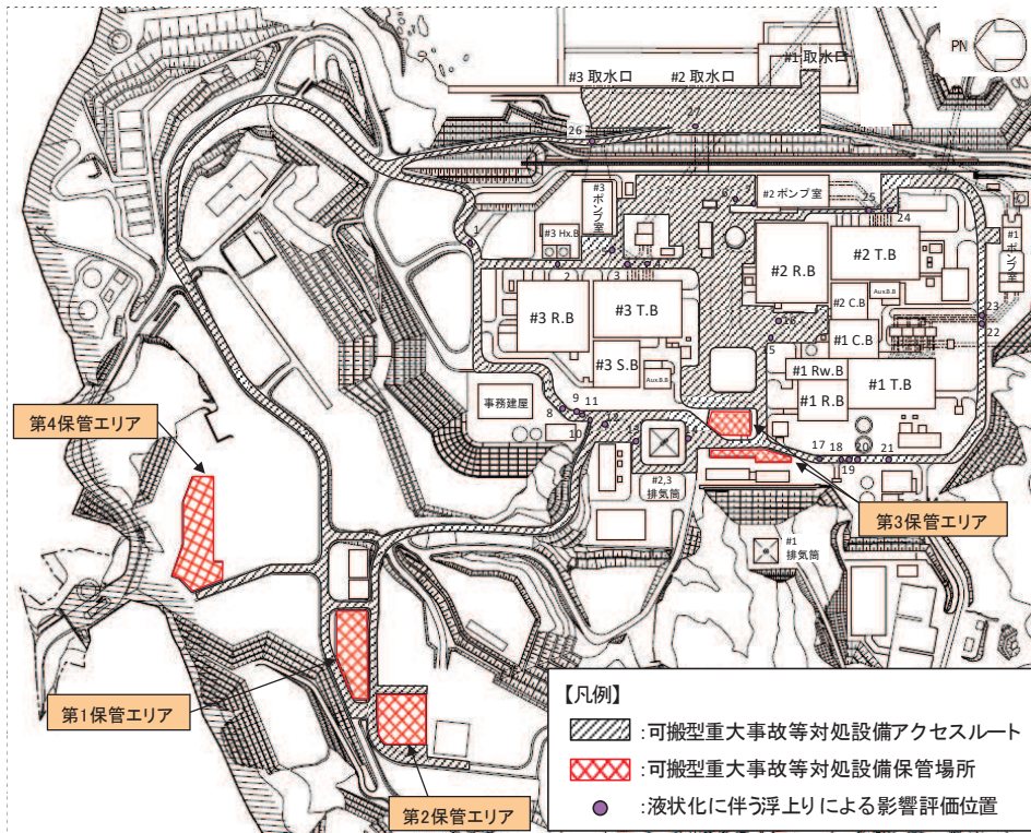
浮上り評価位置
