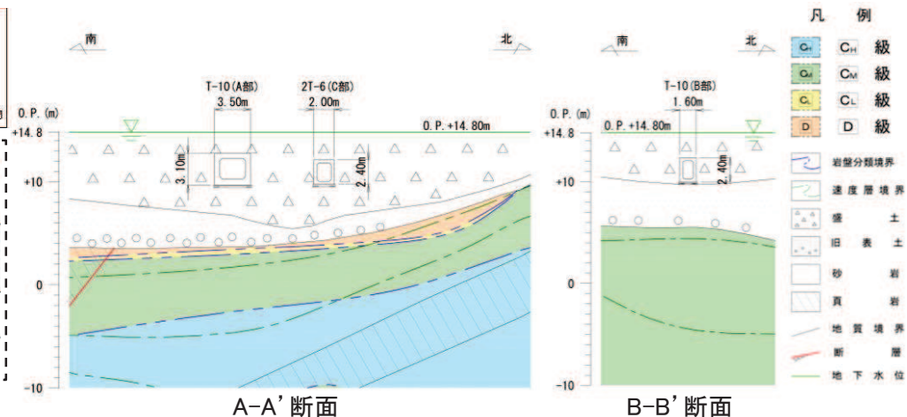
一次元有効応力解析により詳細評価を実施する構造物
