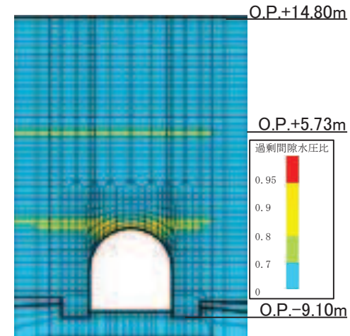
断面①
