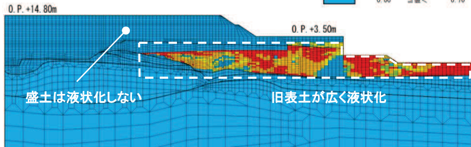
検証解析における最大過剰間隙水圧比分布(液状化強度特性:下限値)
