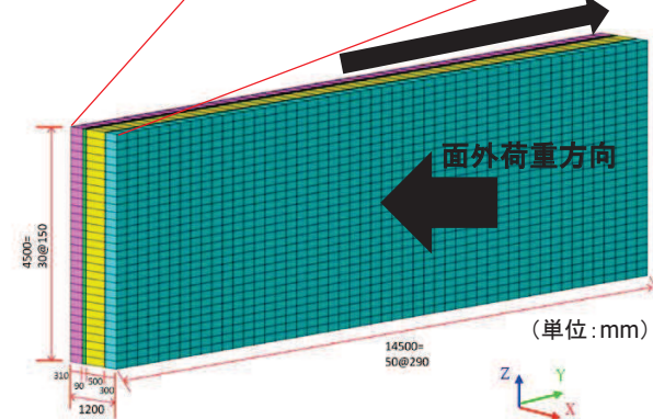
数値解析モデル
