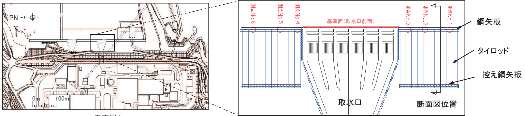
平面図*
