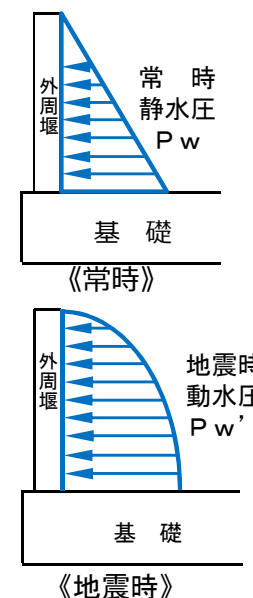
■ 検討断面モデル
