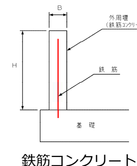
■ 構造概略断面図
