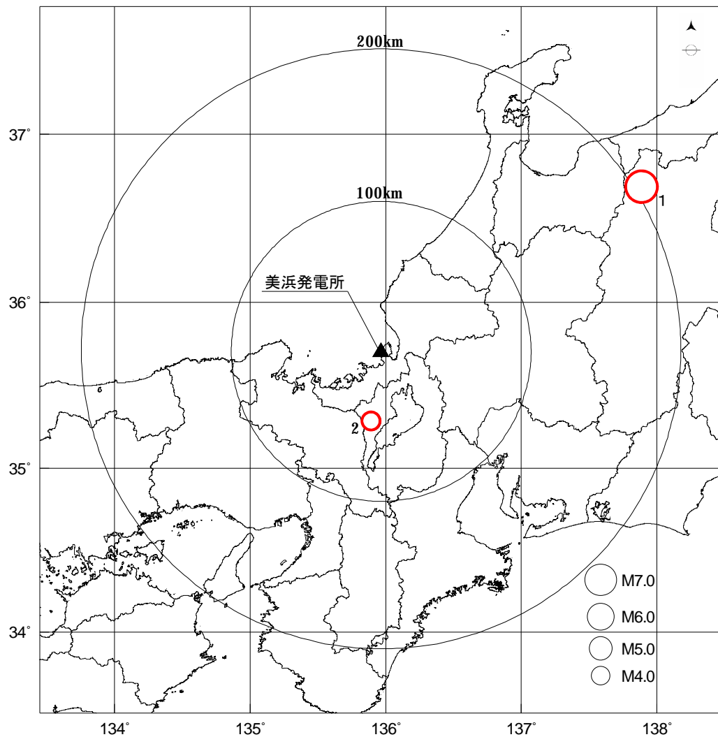
敷地で観測された主な地震の震央分布
