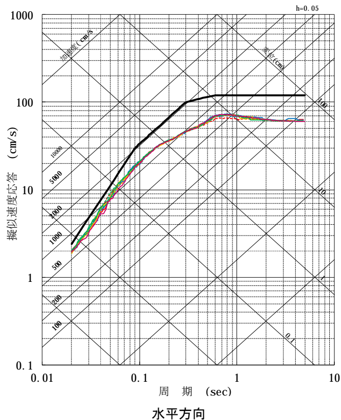
【参考】標準応答スペクトル(地盤増幅特性考慮)と美浜発電所の基準地震動Ss-1との比較
