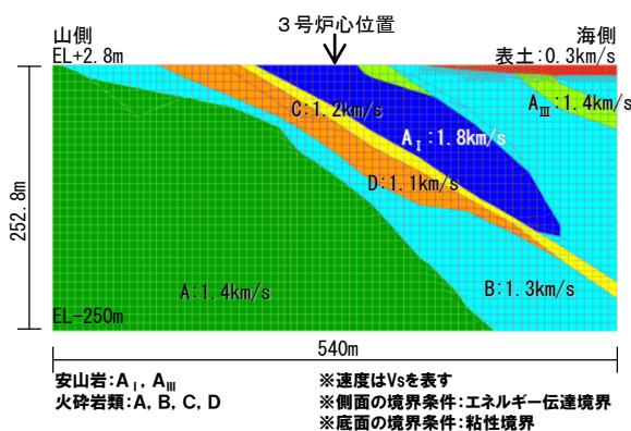
3号炉地盤モデル(最大傾斜断面)
