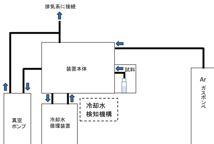
系統図
