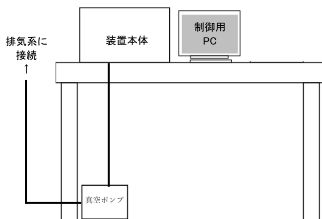
系統図
