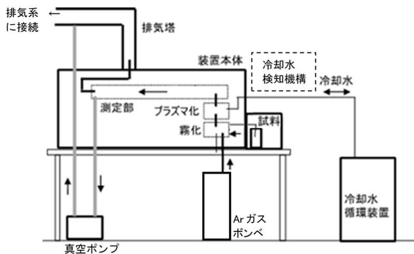
系統図
