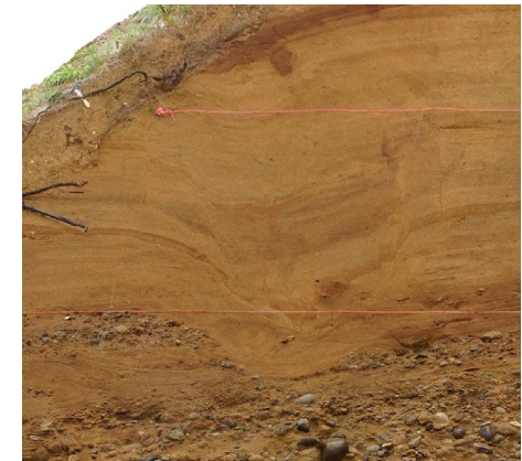
正断層構造を形成する断裂群(④) 拡大写真
