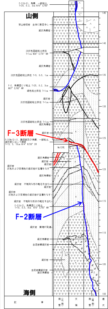
F-2断層とF-3断層の切りあい部の試掘坑スケッチに加筆 (G坑始点からの距離100.0~144.2m)
