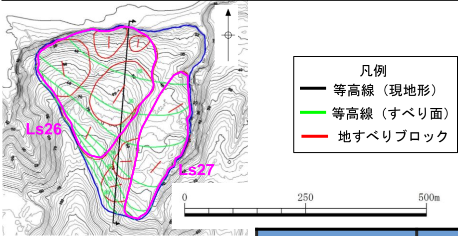
すべり面 (Ls26+27)
