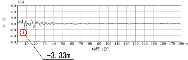
2号炉取水口(東) (最大水位下降量-3.33m+期望平均干潮位T.P.-0.02m -地盤変動量0.34m≒T.P.-3.7m)
