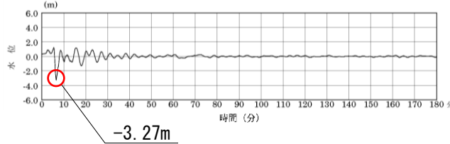
2号炉取水口(西) (最大水位下降量-3.27m+期望平均干潮位T.P.-0.02m -地盤変動量0.34m≒T.P.-3.7m)
