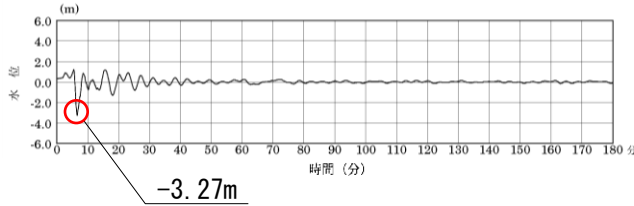
2号炉取水口(西) (最大水位下降量-3.27m+期望平均干潮位T.P.-0.02m -地盤変動量0.34m≒T.P.-3.7m)
