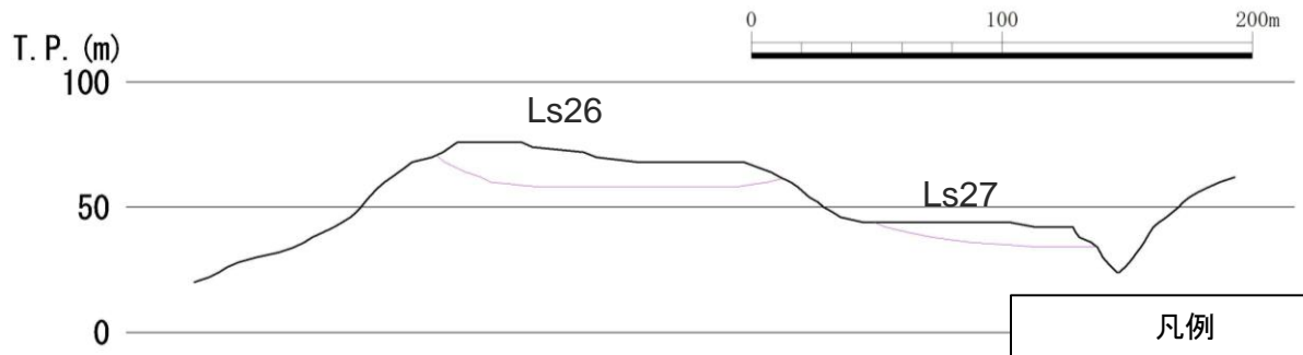
断面図 (Ls26及びLs27の横断方向)
