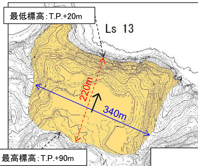
平面長さ・幅の設定
