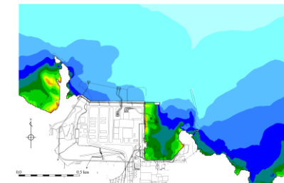
基準津波2, 日本海東縁部 (2領域連動モデル: 防波堤有り)
