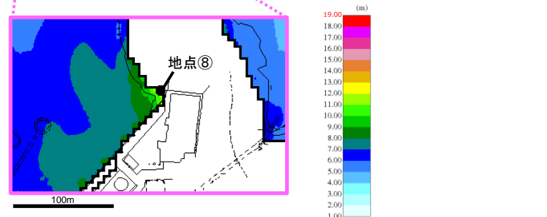
基準津波1, 日本海東縁部 (鳥取県モデル: 防波堤無し)
