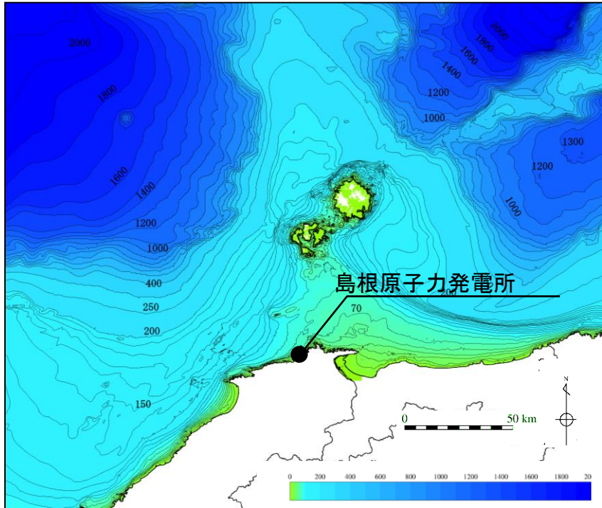
海底地形
