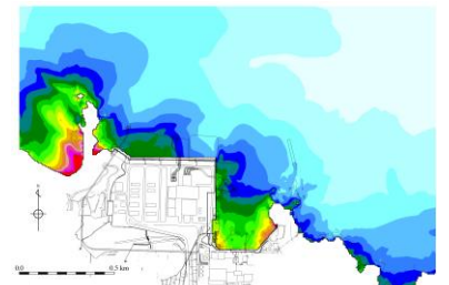
基準津波5, 日本海東縁部 (2領域連動モデル: 防波堤無し)
