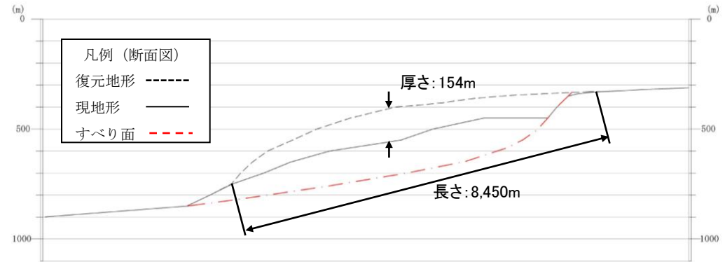
断面図
