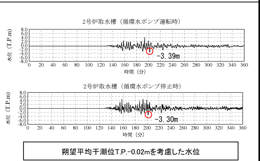
2号炉取水槽での水位の時刻歴波形※
