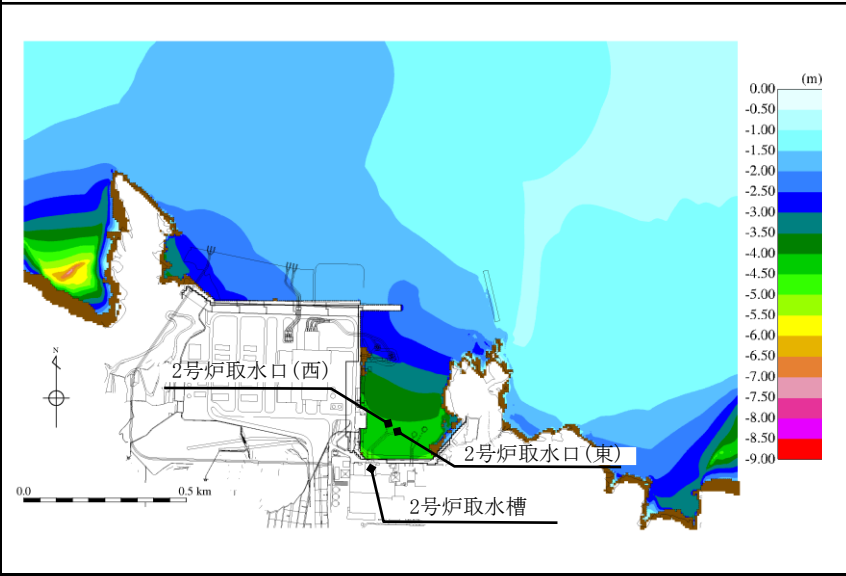
最大水位下降量分布
