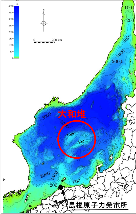
海底地形
