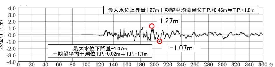
基準津波4
