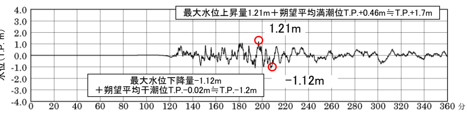
基準津波3
