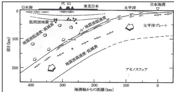
図3.6 東北日本の地殻・上部マントルの東西鉛直断面模式図(Hasegawa et al., 1994) 丸は地震の震源を、震源に付けた矢印は震源に働く力あるいは断層の動きを示す。 ・日本海東縁に沿っては、1983年日本海中部地震、1993年北海道南西沖地震など、逆断層型の大地震が帯状に分布。 ・太平洋側のプレート境界である日本海溝や千島海溝の場合のように、地表面でプレート境界が1本の線で表されるという明確な証拠はみつかっておらず、幅広い帯状の領域で2つのプレートの収束を分担していると考えられる。 ・大陸性地震では、深さ10-15km付近にデタッチメントがあり、それより浅い上部近くに地震の原因となる断層が形成されると考えられている。背斜構造の規模もデタッチメント深度が15km前後であることを支持する。
