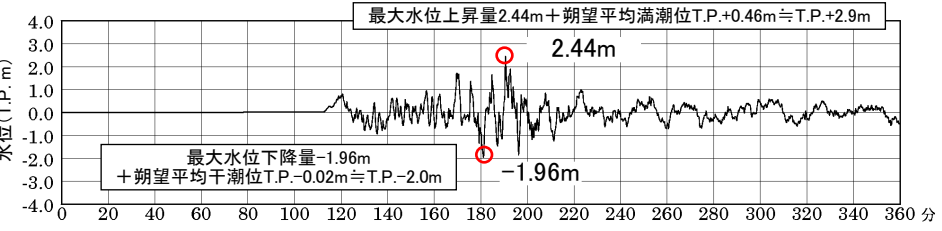
基準津波2
