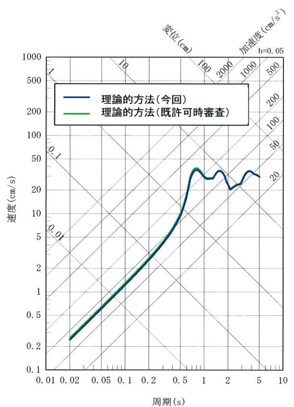
NS方向
