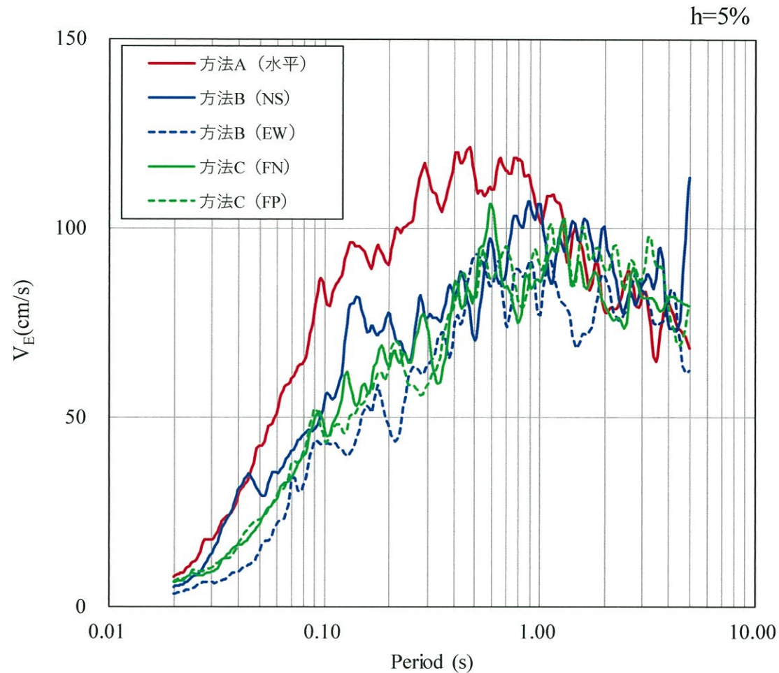
方法A～Cに基づく模擬地震波の入力エネルギースペクトル
