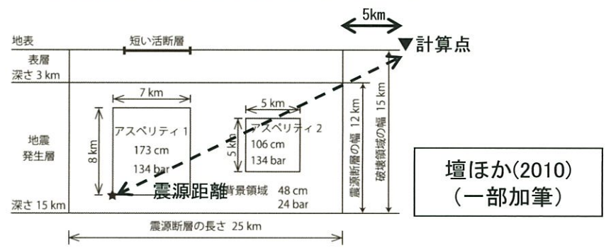
検討に用いた横ずれ断層の震源モデル
