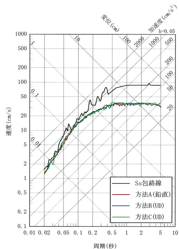
鉛直方向
