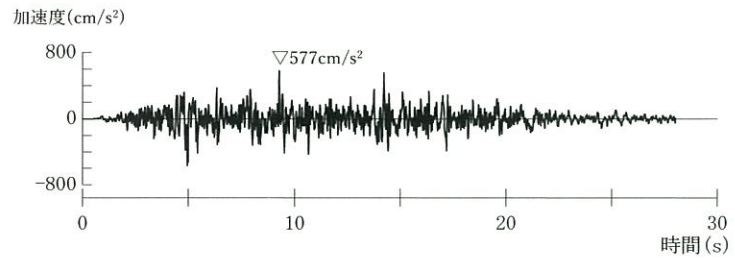
水平方向
