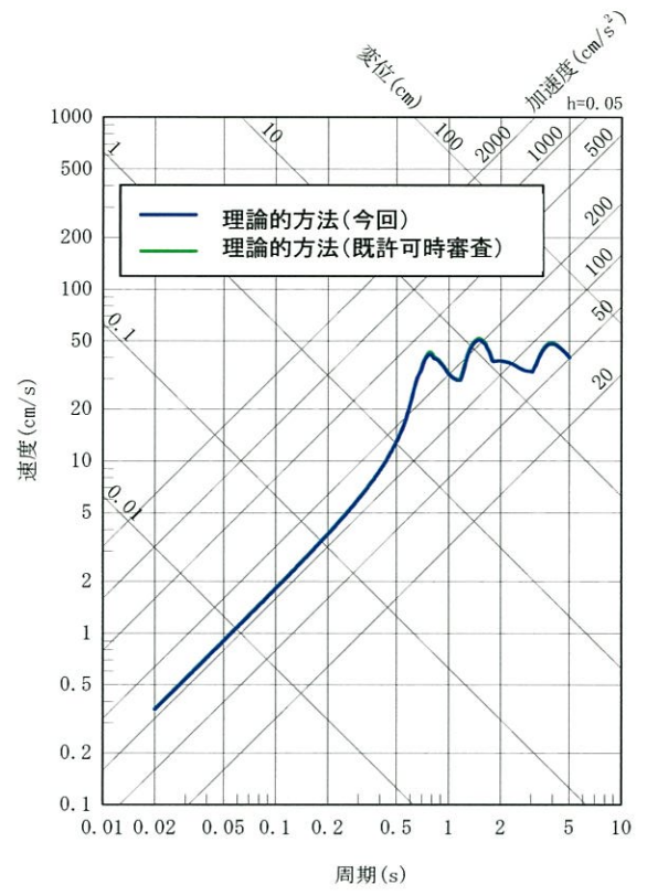
EW方向
