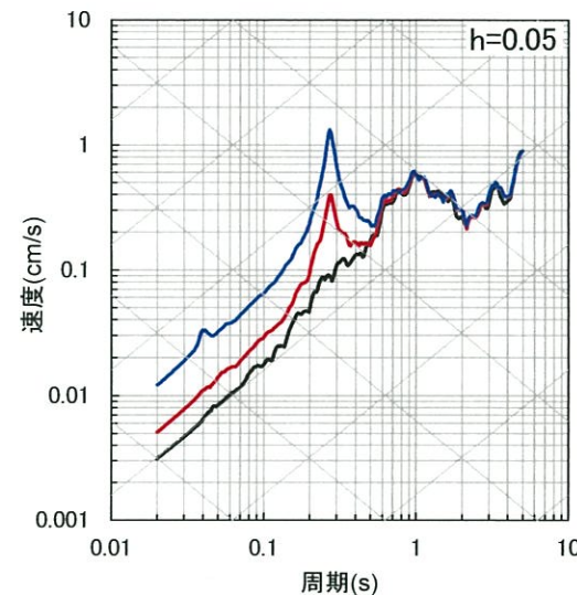
NS方向
