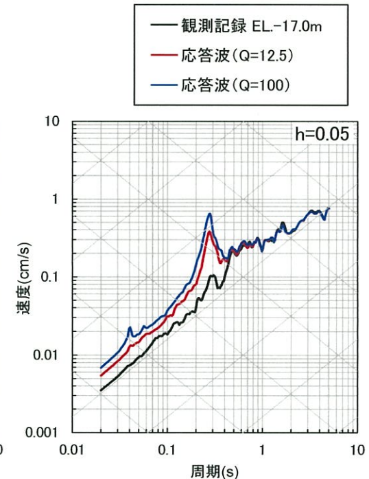
EW方向
