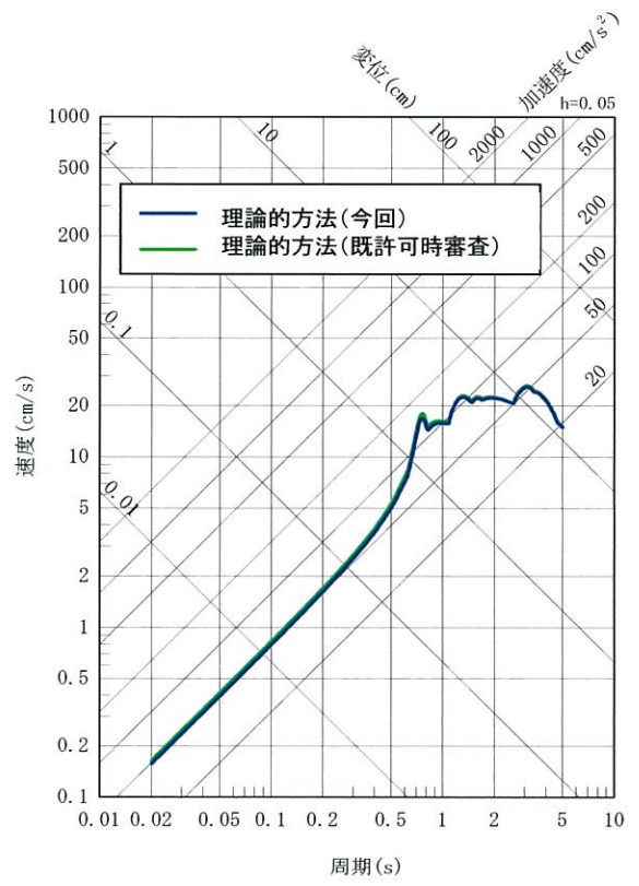
UD方向
