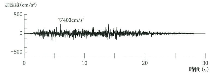
鉛直方向
