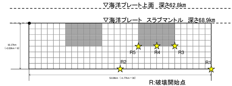
ケース2(地震規模・短周期レベル)
