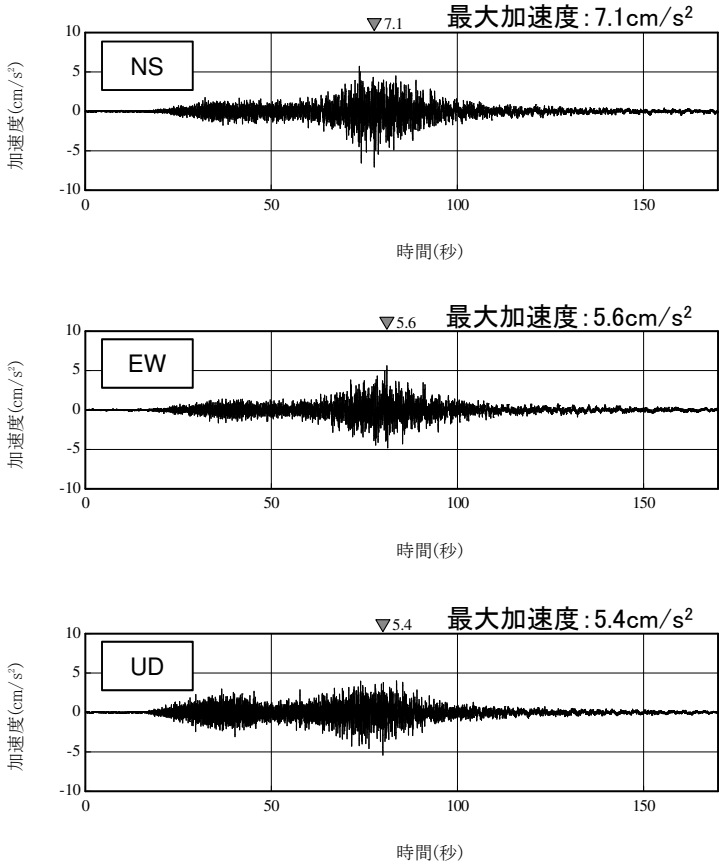
2011年3月11日三陸沖の地震の時刻歴波形 (自由地盤T.P.+2.0m観測点のはざとり波, PN基準)
