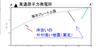
断層配置図(断面)
