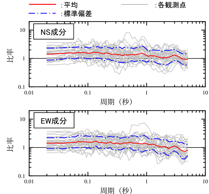
Noda et al.(2002)残差の比(4.7地震/2.13地震)
