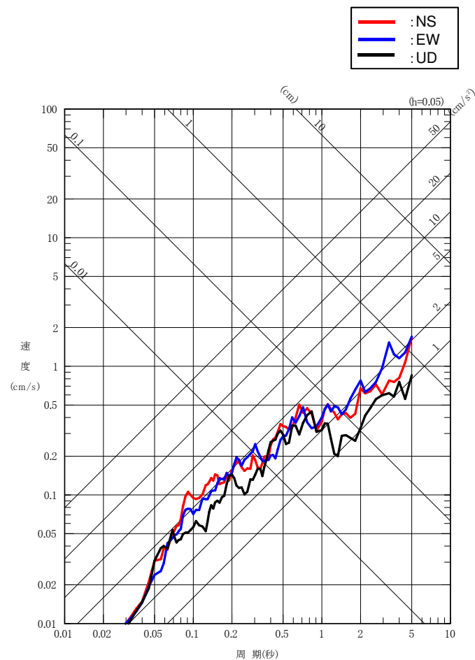
2011年7月10日三陸沖の地震の応答スペクトル (自由地盤T.P.+2.0m観測点のはざとり波, PN基準)
