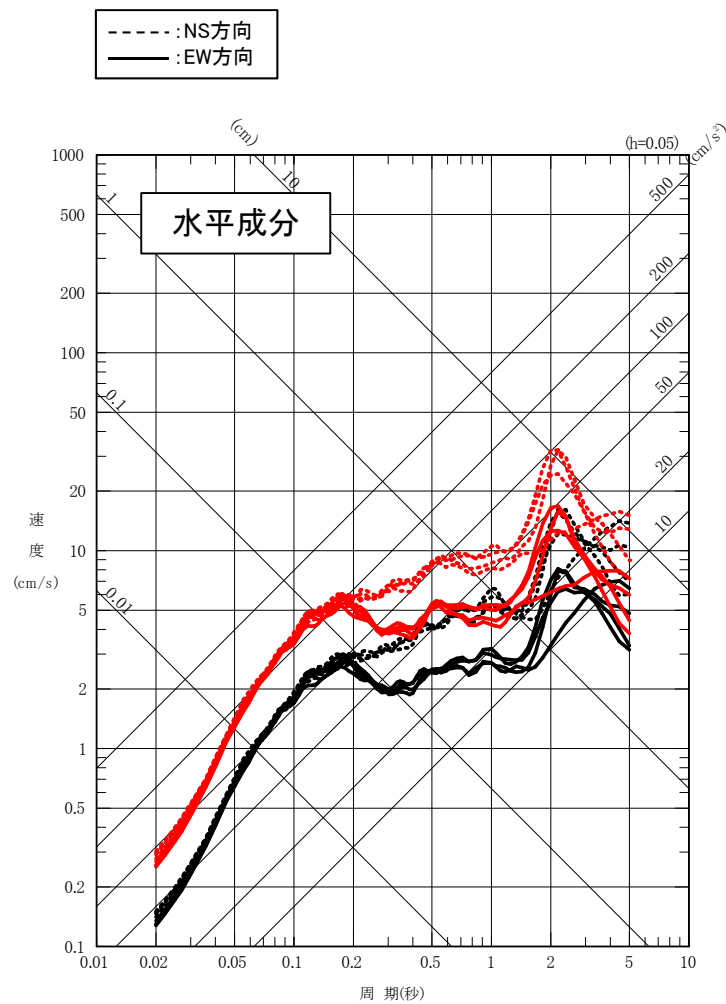
沖合いのやや浅い地震(北海道)(検討対象地震)の地震動評価(平均応答スペクトル)
