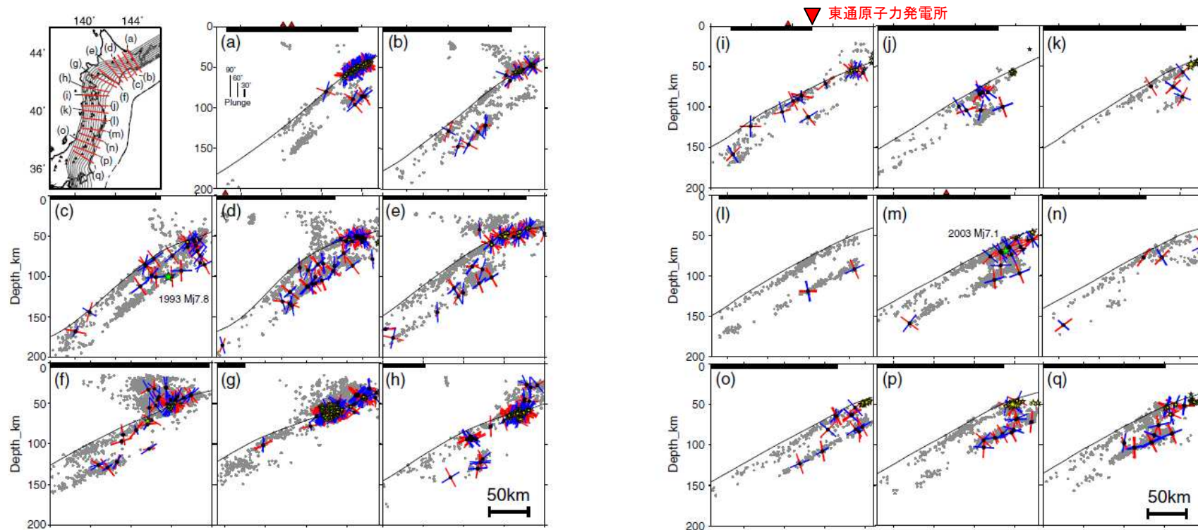
●:各断面から10km以内で発生した地震, 青線:T軸, 赤線:P軸, ☆:繰返し地震 ●:プレート境界で発生した低角逆断層地震, 黒線:プレート上面
