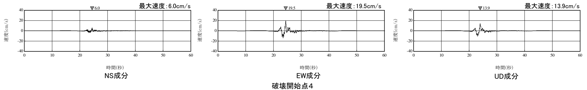
敷地下方DC型地震のうちケース1(基本ケース)の速度波形(PN基準)
