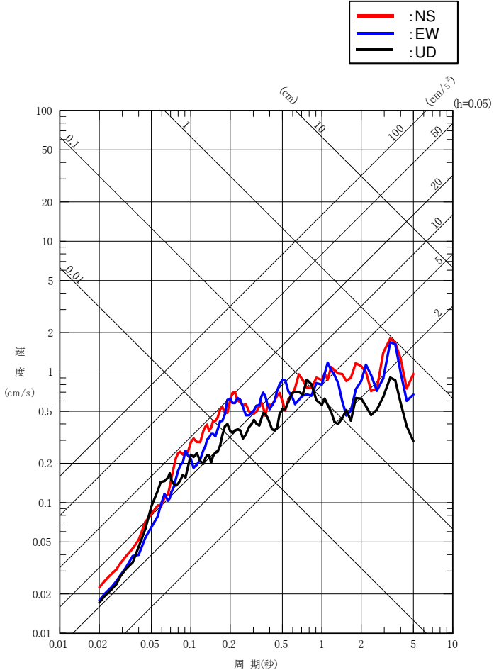
2011年3月11日三陸沖の地震の応答スペクトル (自由地盤T.P.+2.0m観測点のはざとり波, PN基準)
