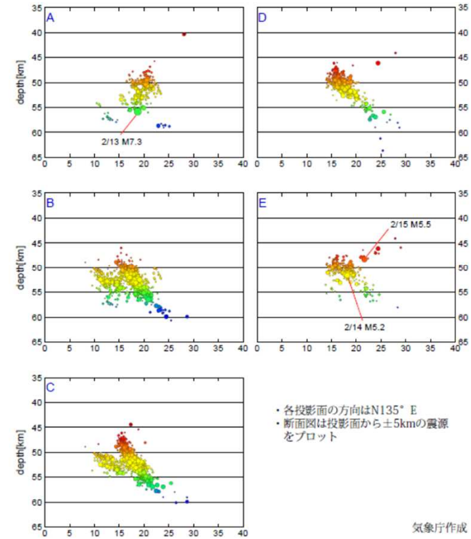
断面図
