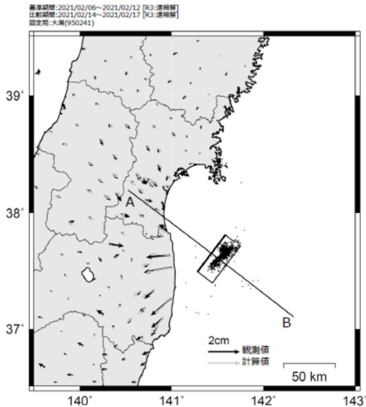
南東傾斜の断層モデル
