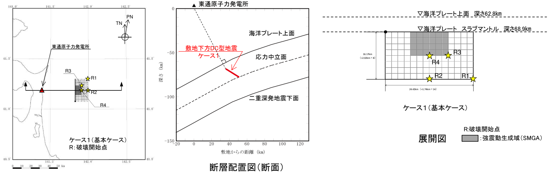
断層配置図
