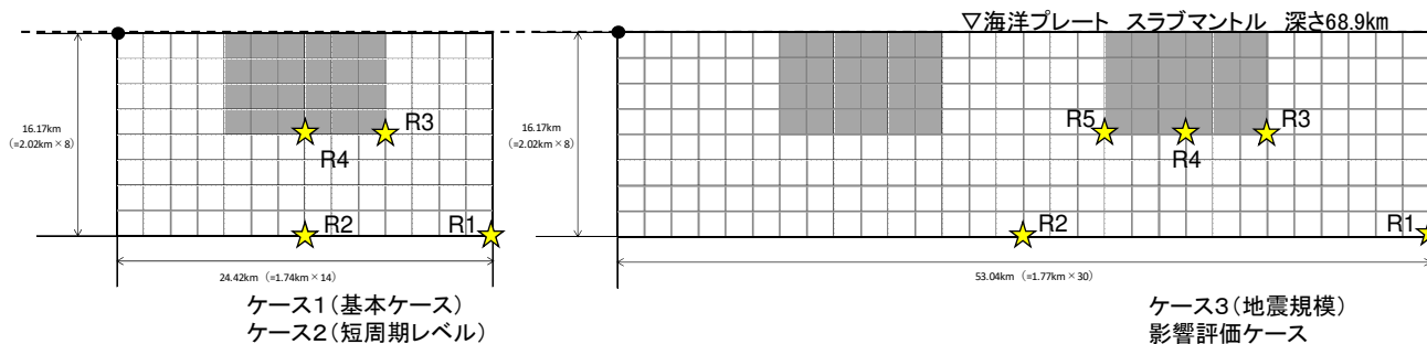
敷地下方DC型地震 展開図
