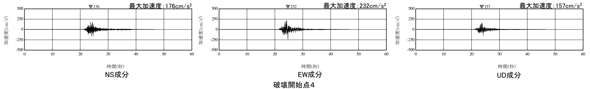
敷地下方DC型地震のうちケース1(基本ケース)の加速度波形(PN基準)
