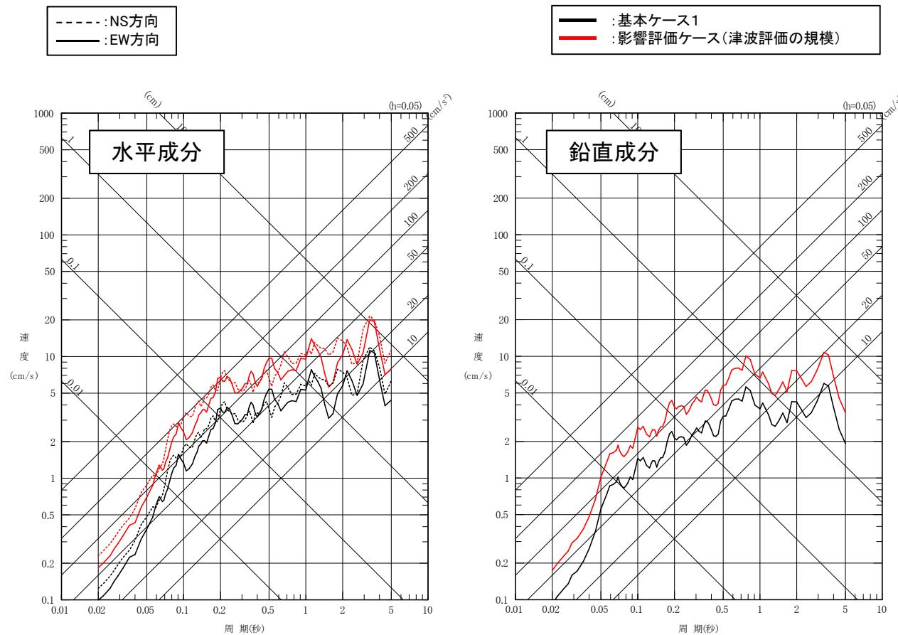
アウターライズ地震 (検討対象地震) の地震動評価 (PN基準) アウターライズ地震の応答スペクトル = 観測記録の応答スペクトル × Noda et al.(2002)の比率
