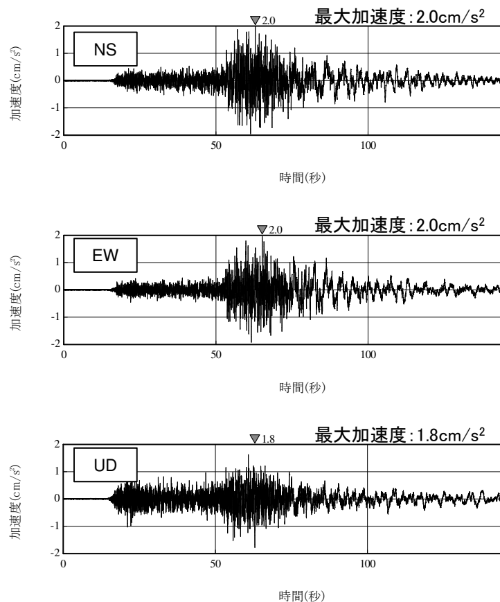
2011年7月10日三陸沖の地震の時刻歴波形 (自由地盤T.P.+2.0m観測点のはざとり波, PN基準)
