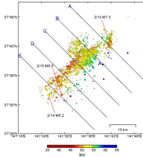
震央分布
