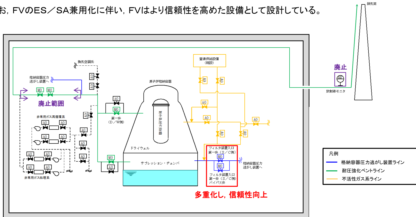
第7図 耐圧強化ベントの廃止範囲
