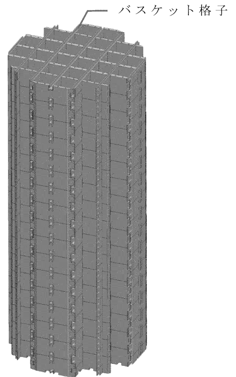
(2) バスケット格子全体図
