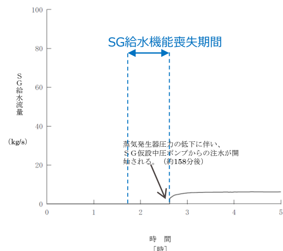
図3 SG給水流量
